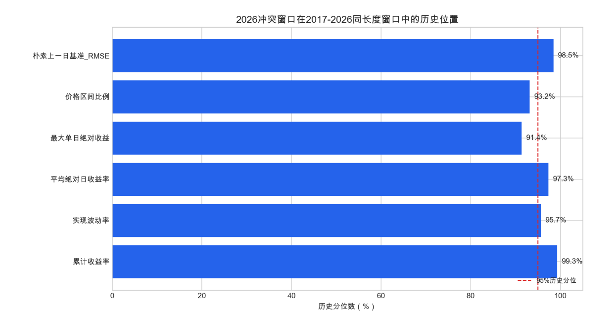
图 32 2026 冲突窗口在历史同长度窗口中的极端性。累计涨幅、波动率和朴素基准误差均处于历史高分位。
