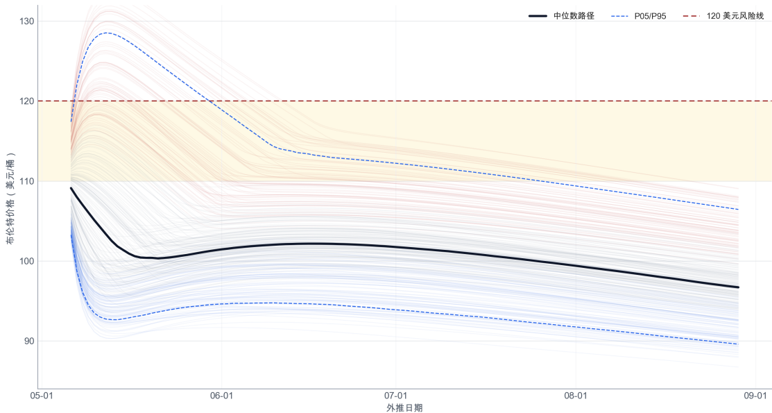
图 26 传统蒙特卡洛路径云图。图中从 2000 条模拟路径中分层抽取代表路径，黑线为中位数路径，蓝色虚线为 P05/P95 条件边界，红色虚线为 120 美元/桶风险线。
