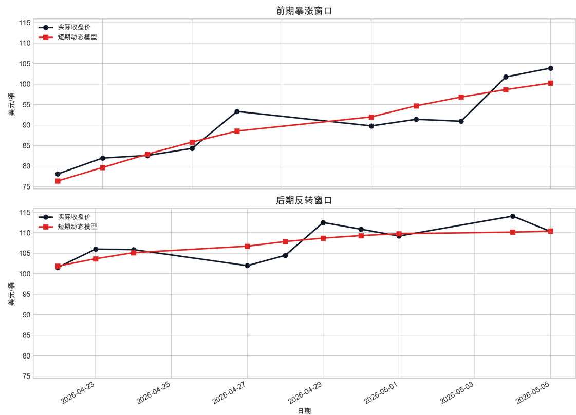
图 17 短期模型拐点局部检验。图中放大前期暴涨窗口和后期反转窗口，用于检查模型是否慢半拍跟随真实价格。
