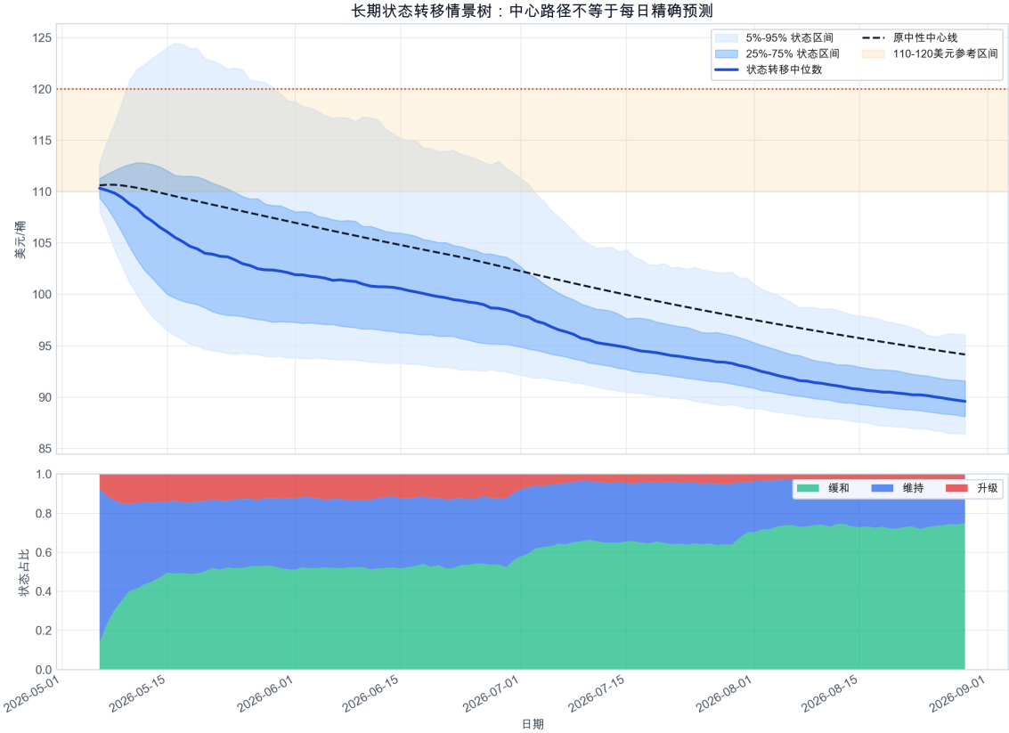
图 22 长期状态转移情景树。上图为状态转移后的价格扇形区间，下图为缓和、维持、升级三类状态的样本占比；该图用于回应长期中性线过平的问题，并展示二次升级风险如何进入尾部区间。
