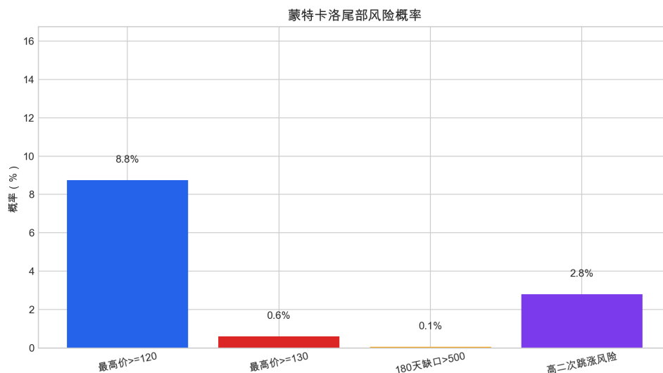
图 25 蒙特卡洛尾部风险概率。
