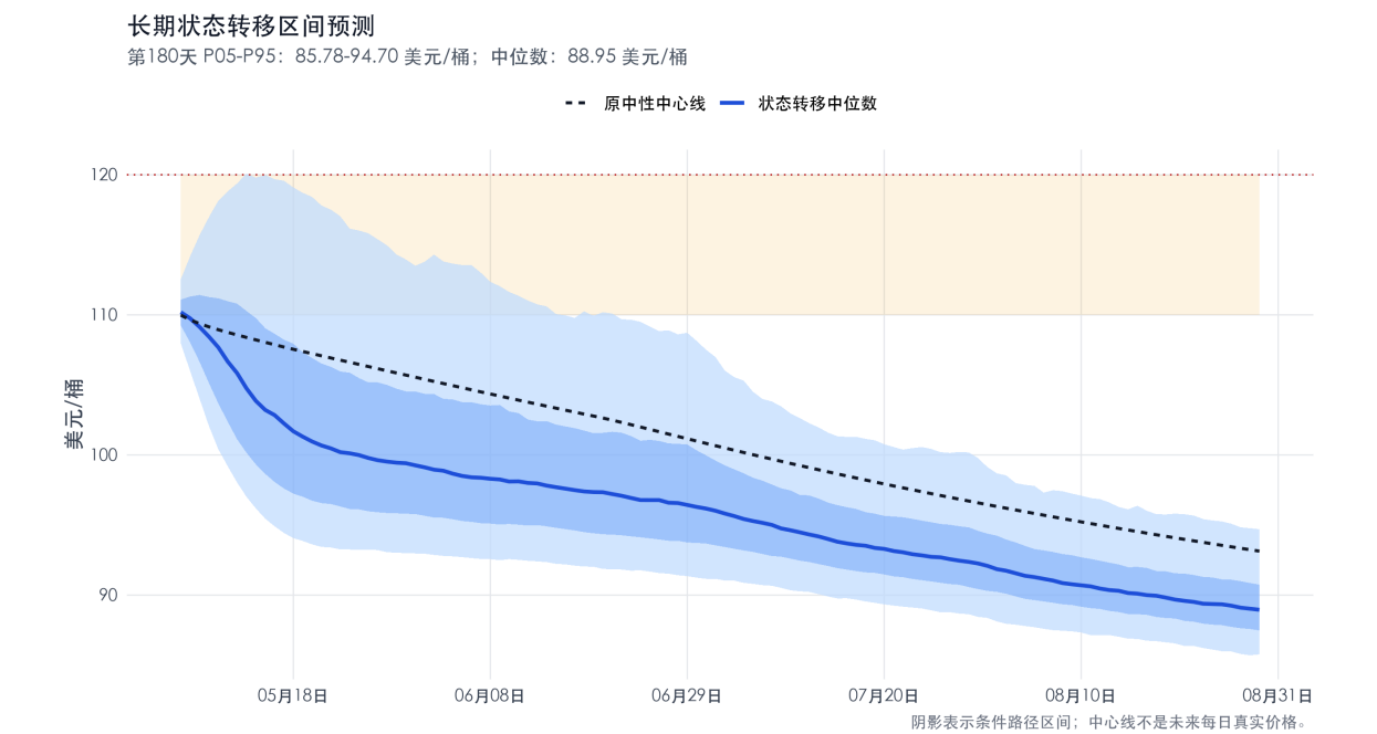
图 26 R/ggplot2 长期状态转移区间预测。双层阴影分别表示 5%–95% 和 25%–75% 条件区间，虚线为原中性中心路径。
