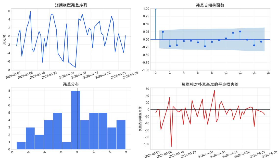
图 16 短期模型统计审计。图中展示残差序列、残差自相关、残差分布和相对朴素基准的平方损失差。
