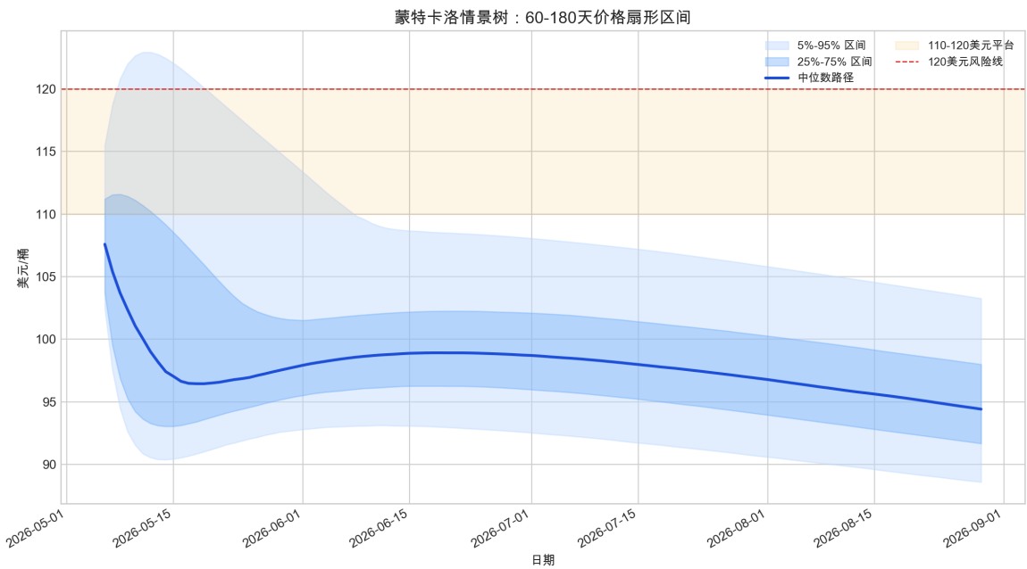
图 20 长期情景预测主图：蒙特卡洛情景树价格扇形区间。深色区间为 25%–75%，浅色区间为 5%–95%。三情景中心路径应与该区间共同解读。
