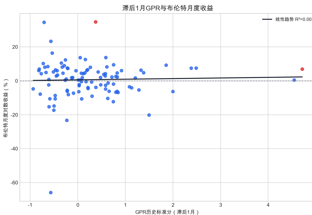
图 28 滞后 1 月 GPR 与布伦特月度收益关系。散点关系较弱，说明 GPR 更适合作为风险溢价外部审计，而非单独点预测模型。
