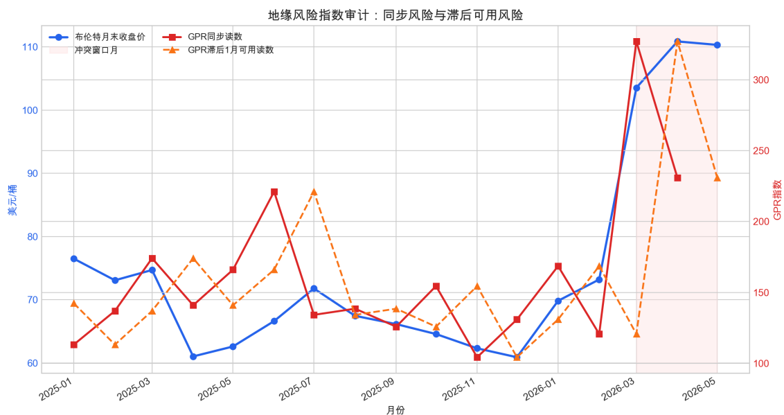
图 27 地缘风险指数审计：同步 GPR 与滞后可用 GPR。3 月油价解释不能使用 3 月同步 GPR，4 月以后才可使用已实现的 3 月风险读数。
