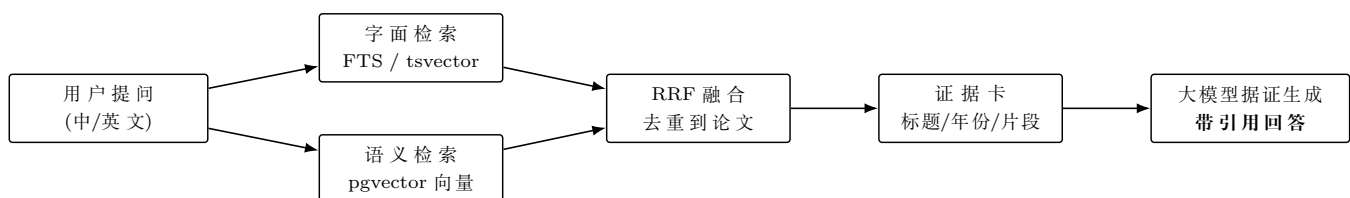
图 2 混合检索 + 证据接地生成链路 (中文问句可跨语言命中英文文献)
