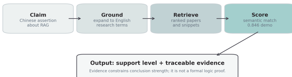
图 9 verify_claim 论断接地流程。数据来源: 工具契约与黄金会话; 输出为支持等级和可追溯证据。
