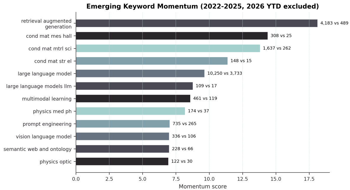
图 9 融合主题词近期动量。数据来源: data/analysis/keyword_trends.csv ; 该指标比较 2024–2025 与 2022–2023 的相对变化, 不把 2026 年末完整数据纳入完整年度动量。
