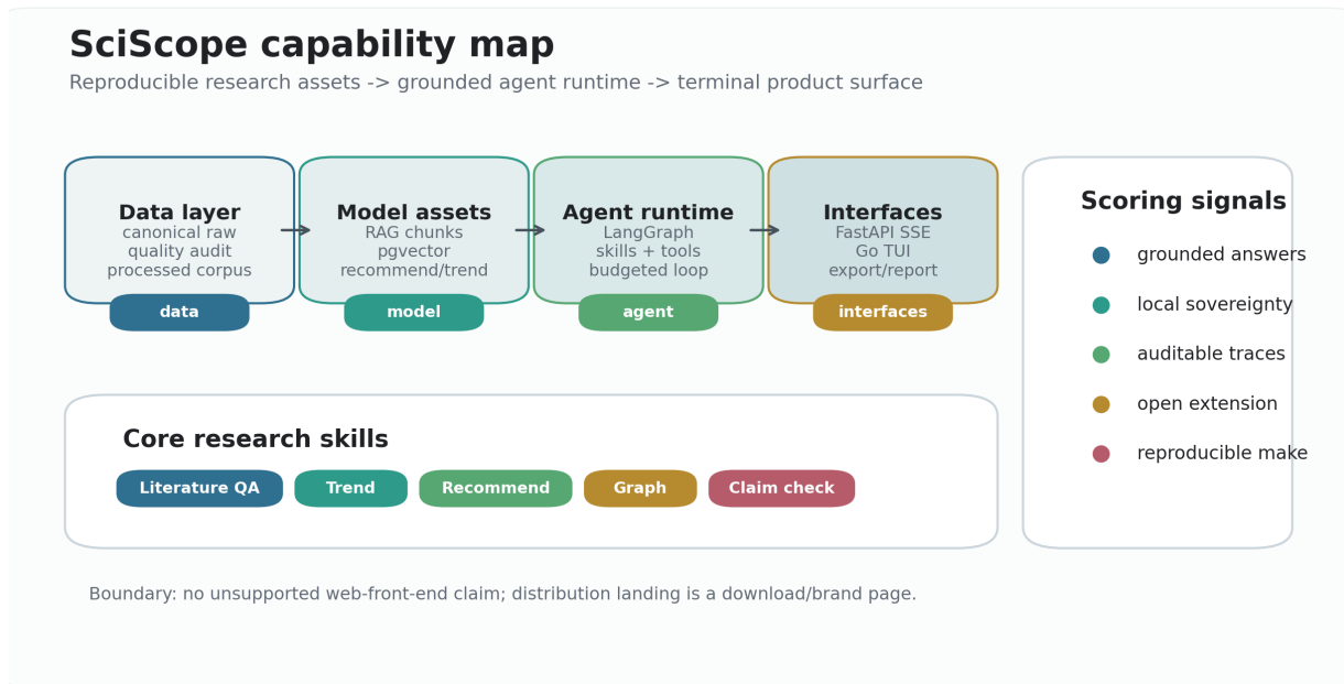
图 2 SciScope 能力地图: 从可复现数据资产到证据接地智能体, 再到终端产品化客户端。数据来源: 系统实现与交付目录映射。
