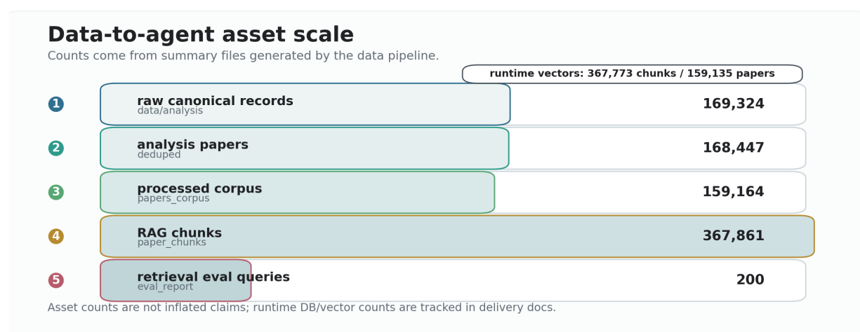
图 7 数据到智能体的资产漏斗。数据来源:data/analysis/summary.json、data/processed/*.summary.json 与 output/eval/eval_report.json; 图中为文件资产口径, 运行时数据库/向量表口径在本章表格中另列。
