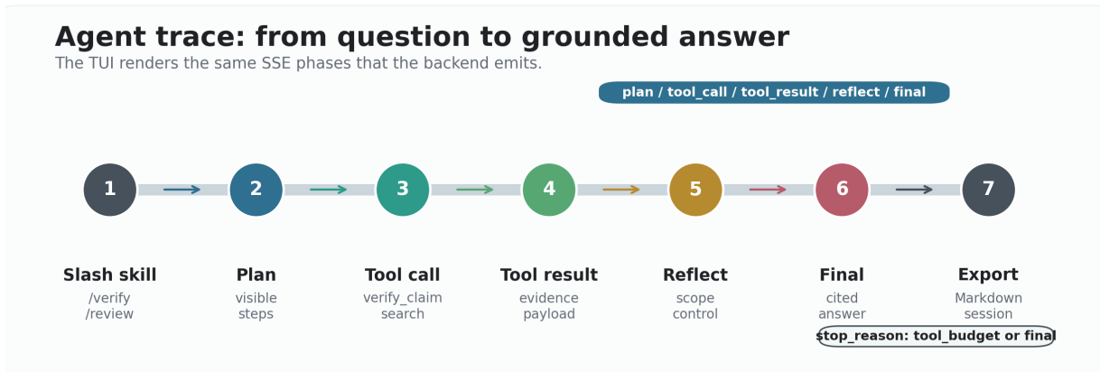
图 5 TUI 中可见的智能体执行轨迹: 科研工作流阶段、工具调用、证据卡、reflect 与 final 均通过 SSE 事件流呈现, 便于评委复核系统不是黑盒问答。
