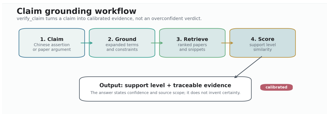
图 9 verify_claim 论断接地流程。数据来源: 工具契约与黄金会话; 输出为支持等级和可追溯证据。
