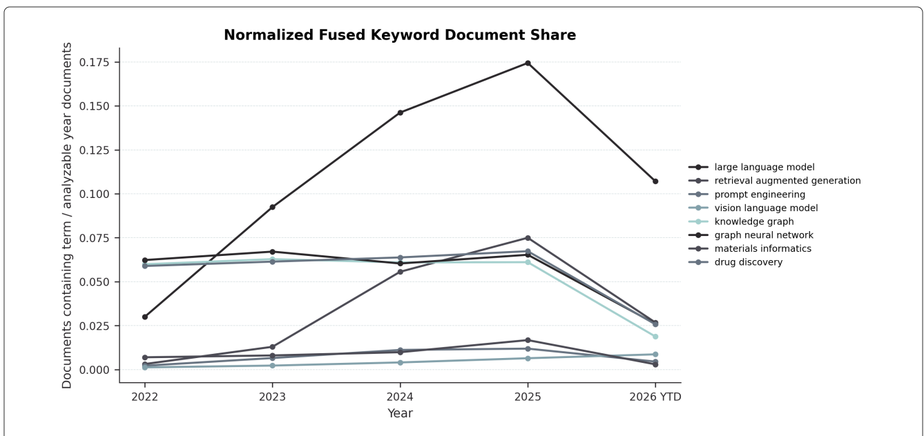
图 10 代表性融合主题词年度归一化文档占比。数据来源: data/analysis/keyword_trends.csv; 归一化后仍持续上升的主题更可能反映真实研究关注变化。
