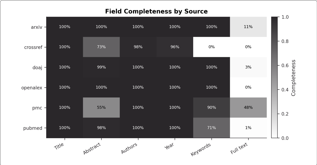
图 2 各来源关键字段完整度矩阵。数据来源: data/analysis/source_quality_report.csv; 颜色越深表示覆盖越高。Crossref 的摘要和关键词覆盖相对较弱, PMC 的正文片段优势明显。
