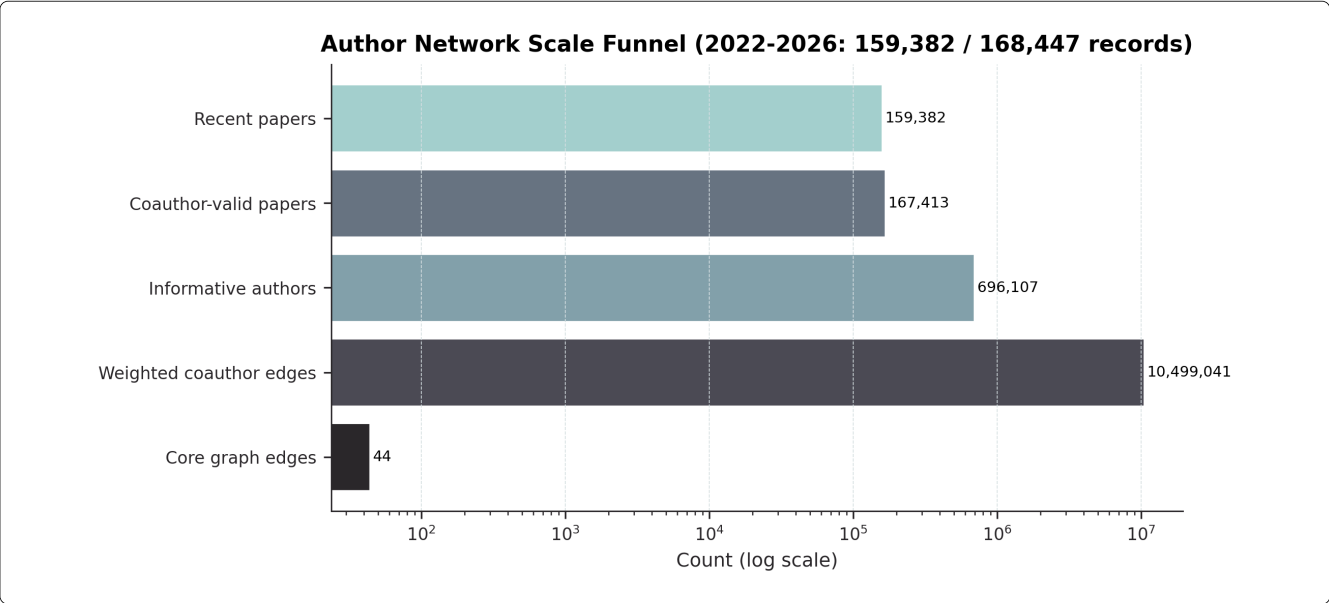
图 15 作者合作网络规模漏斗。数据来源:data/analysis/author_network_diagnostics.csv; 从近五年论文到核心合作图逐步压缩, 以保证网络图具有可读性。
