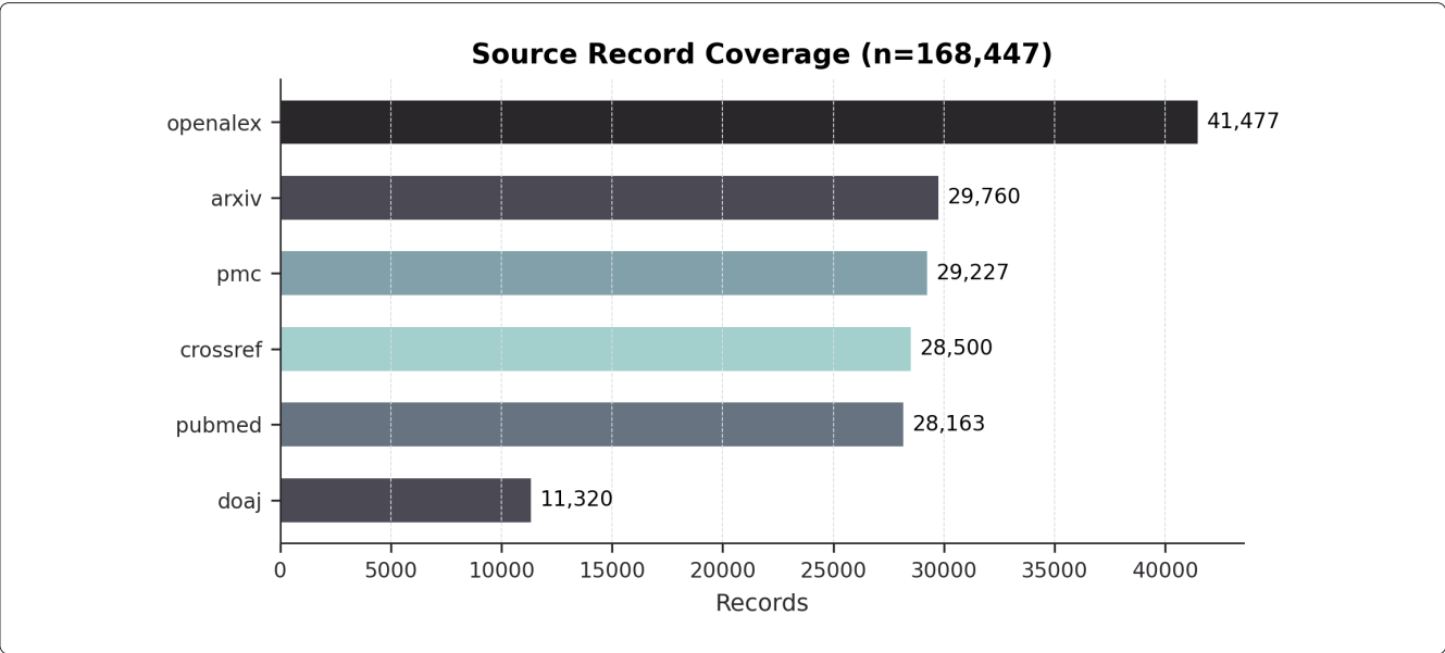
图 1 六个公开来源的标准化分析记录规模。数据来源:data/analysis/source_quality_report.csv; 统计窗口为全分析语料 168,447 条。OpenAlex 规模最大，DOAJ 规模最小，后续跨来源比较需注意来源结构差异。
