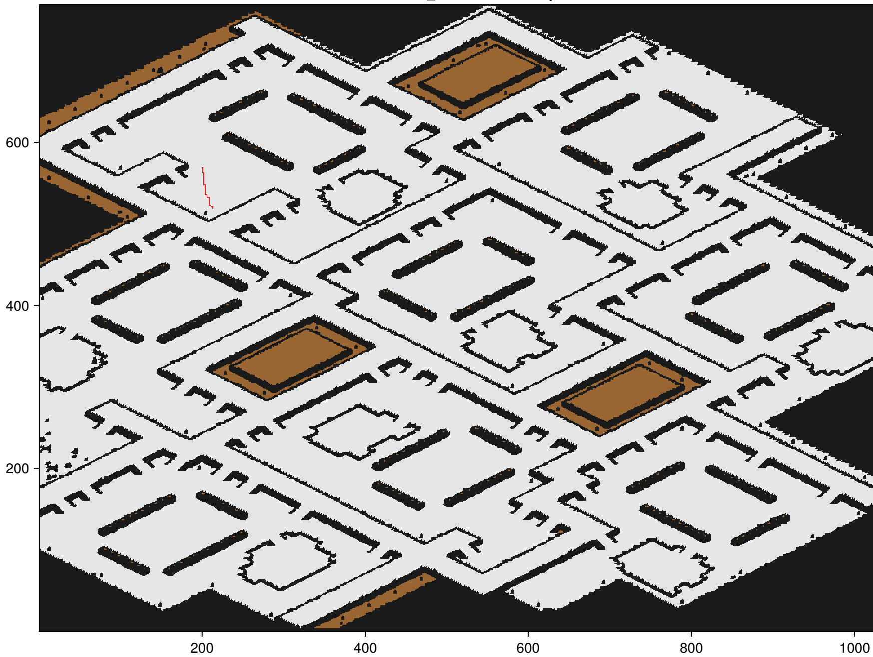
res/Aurora_solutionAstar.map
