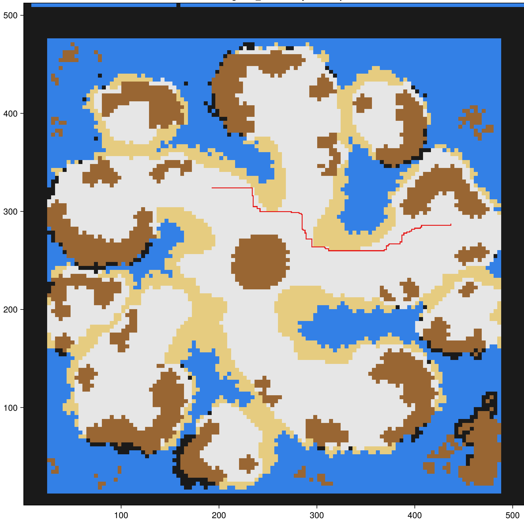
res/theglaive_solutionDijkstra.map
