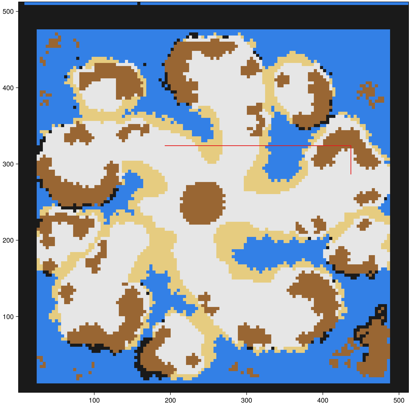
res/theglaive_solutionGlouton.map
