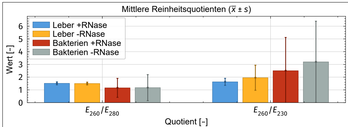
Abbildung 17: Gruppierendes Balkendiagramm der mittleren Reinheitsquotienten E_{260}/E_{280} und E_{260}/E_{230} [-] mit Standardabweichung.
