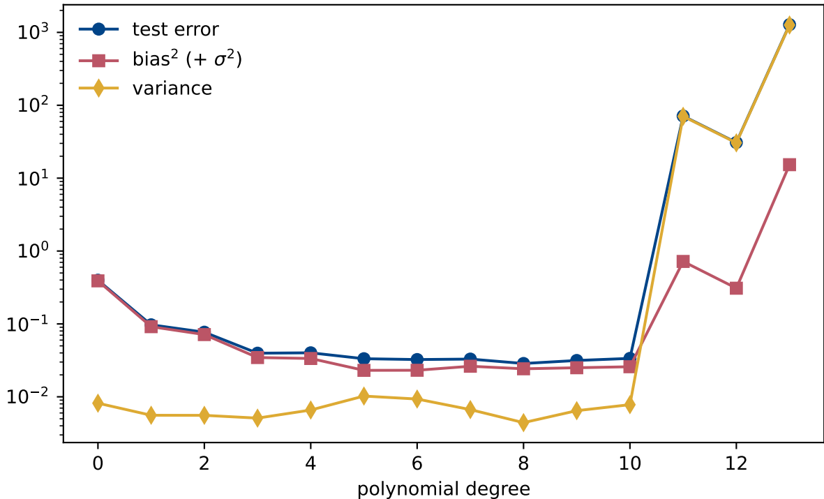
MSE decomposition
