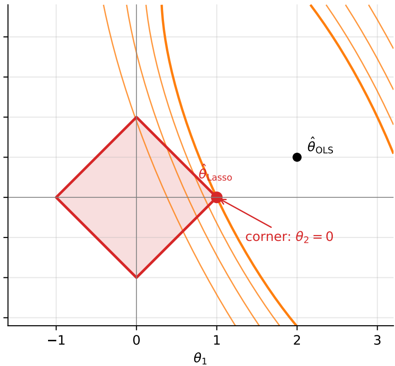
Lasso: |\theta_1| + |\theta_2| \leq t
