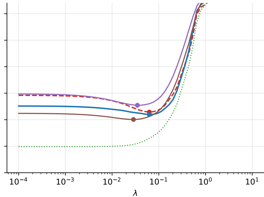
Lasso
