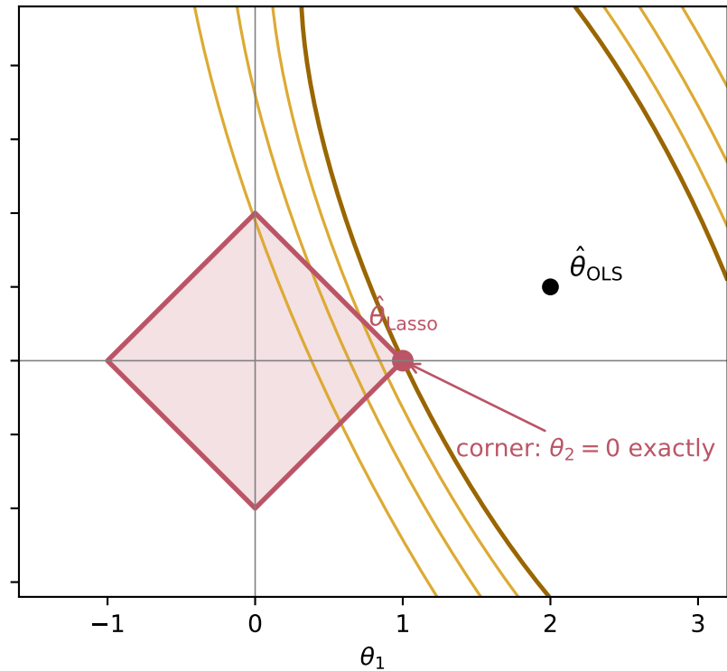
Lasso: |\theta_1| + |\theta_2| \leq t (a rhombus)
