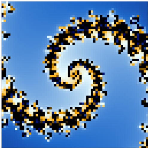
arbitrary precision
