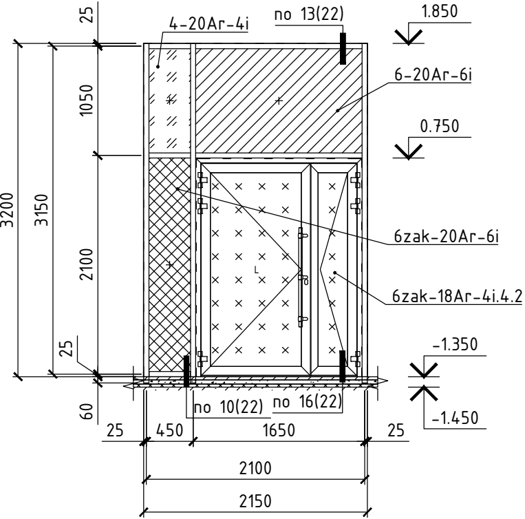
Витраж ВН-3.8 (1 шт.)
