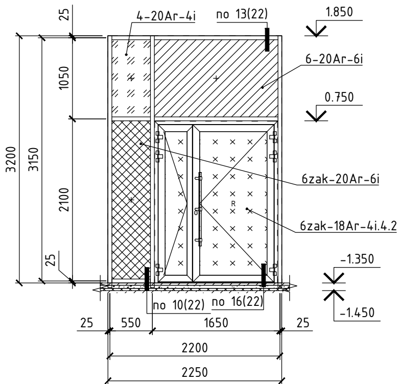
Витраж ВН-3.2 (1 шт.)
