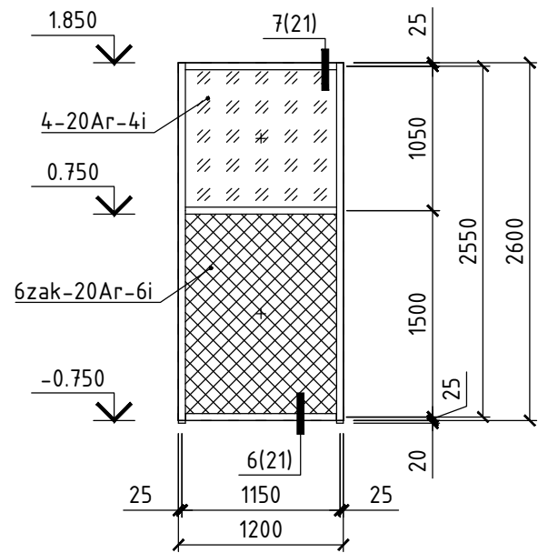
Витраж ВН-1.1 (1 шт.)
