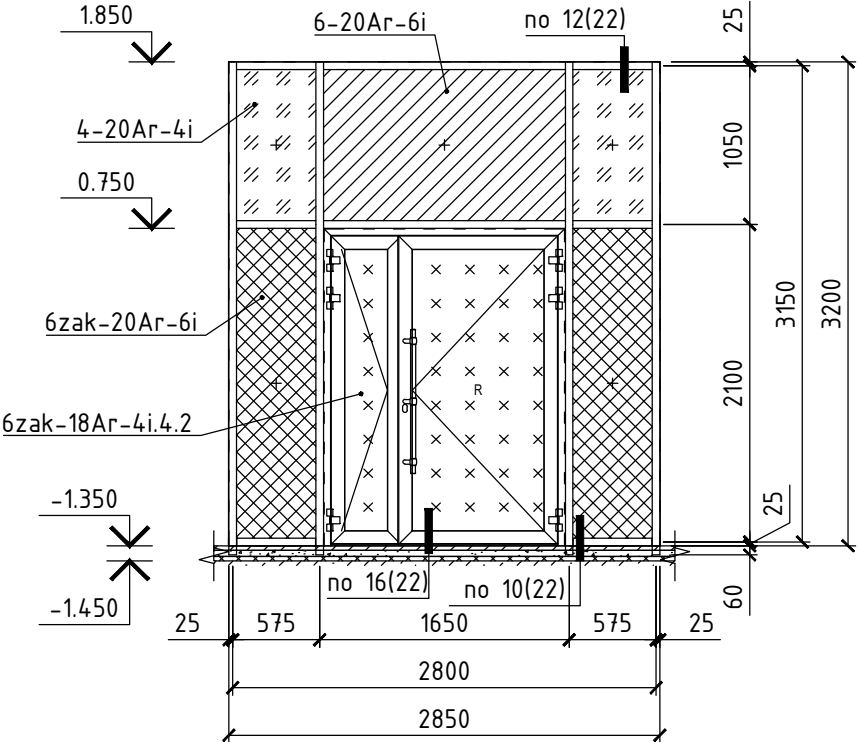
Витраж ВН-3.6 (2 шт.) Козырёк
