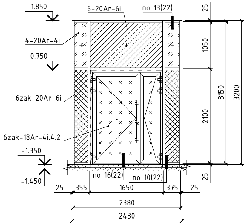
Витраж ВН-2.7 (1 шт.)
