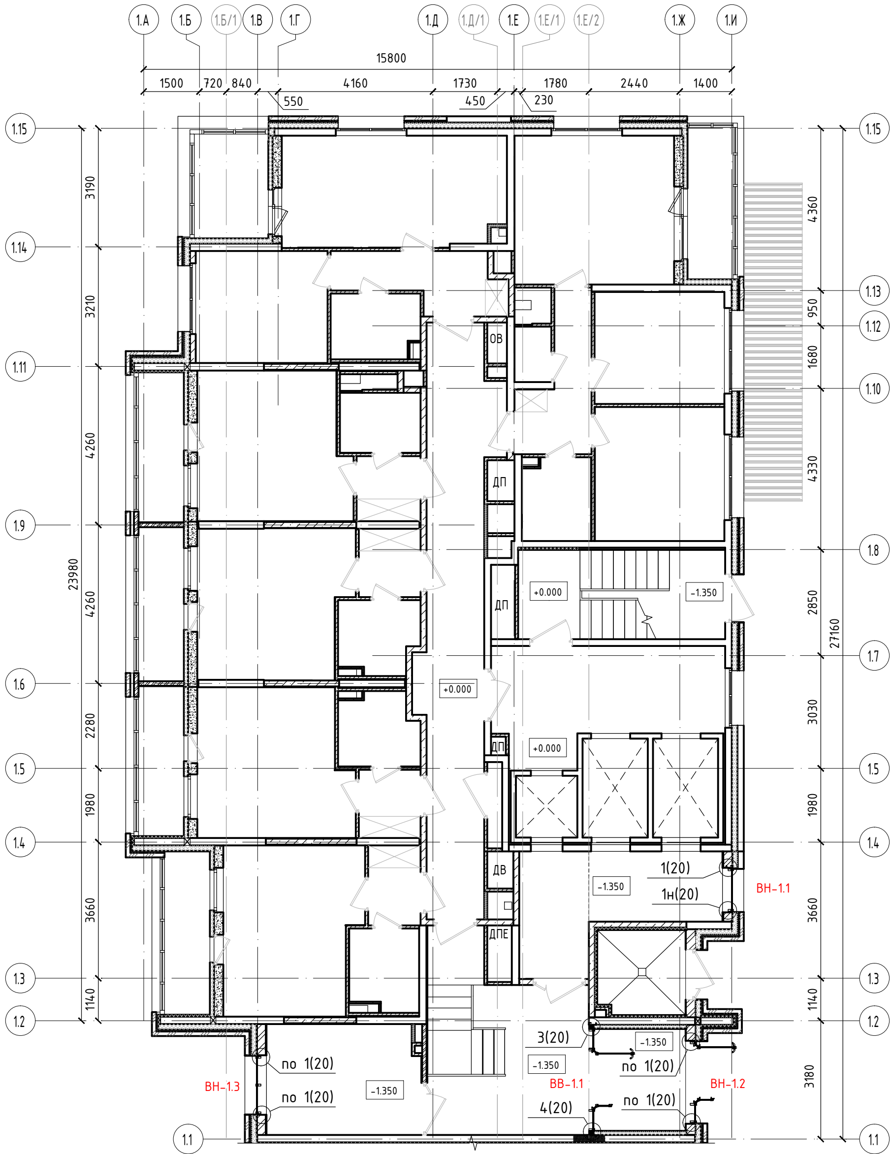
Схема расположения секций
