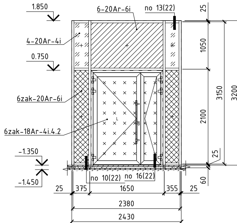
Витраж ВН-3.4 (1 шм.)
