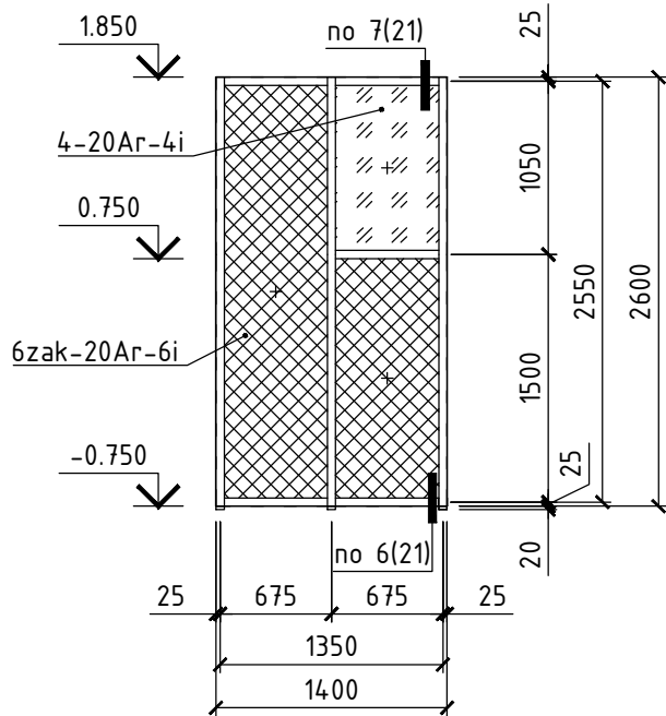
Витраж ВН-2.2 (1 шт.)
