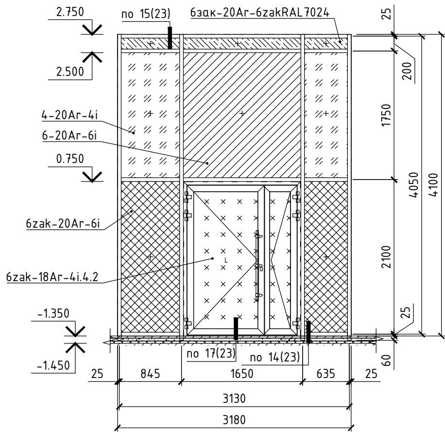
Витраж ВВ-3.2 (1 шт.)
