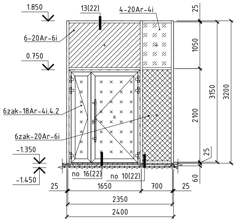
Витраж ВН-2.1 (1 шт.)
