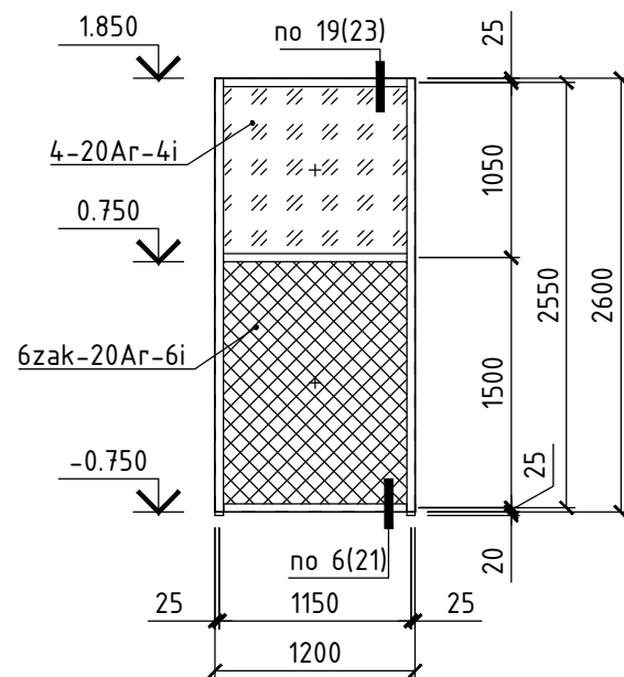
Витраж ВН-3.5 (1 шм.)
