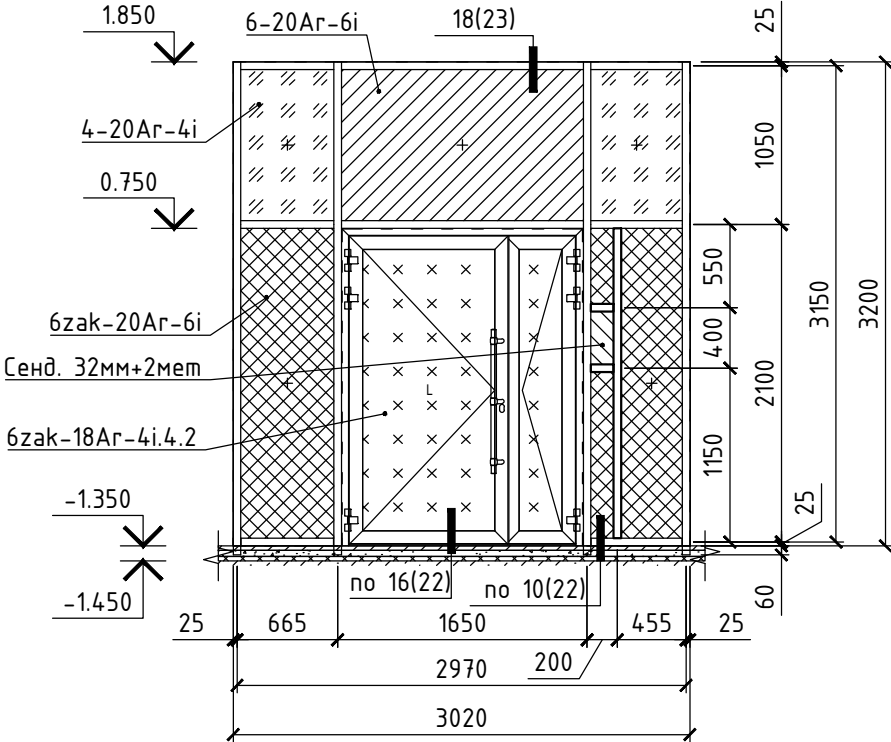
Витраж ВН-3.7 (1 шт.)
