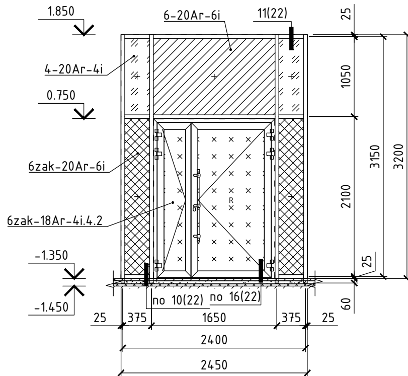
Витраж ВН-3.3 (1 шм.)
