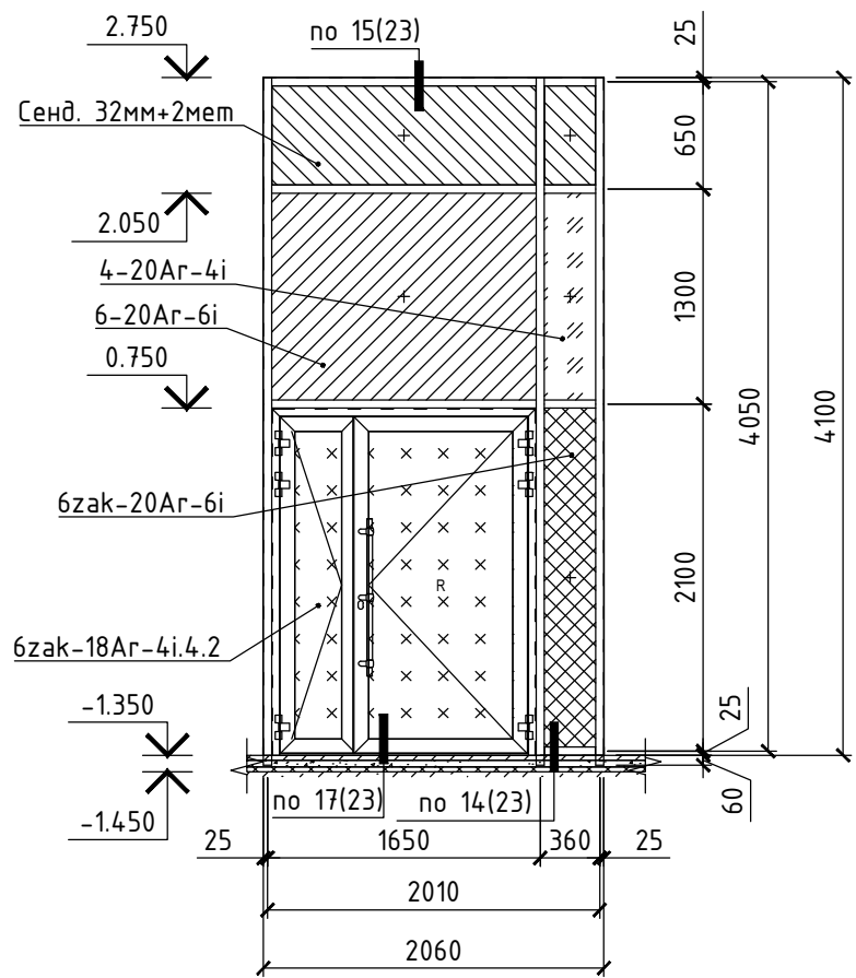
Витраж ВВ-3.1 (1 шт.)
