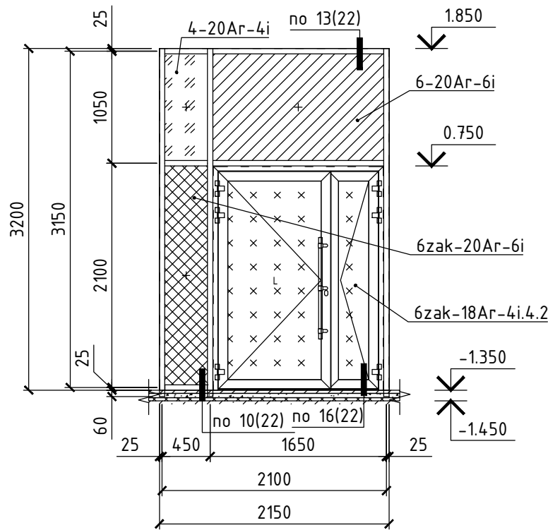
Витраж ВН-4.3 (1 шт.)
