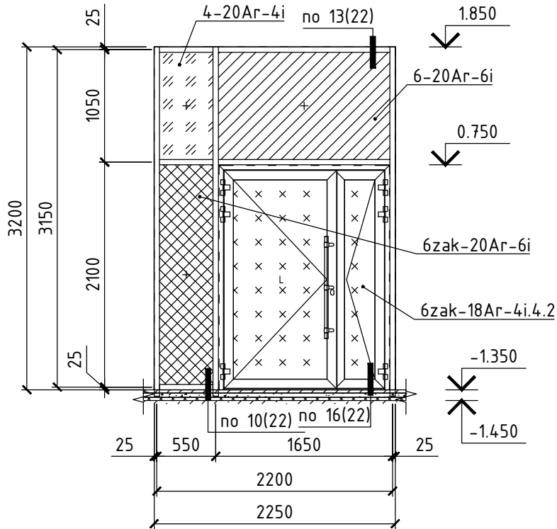
Витраж ВН-4.8 (1 шт.)
