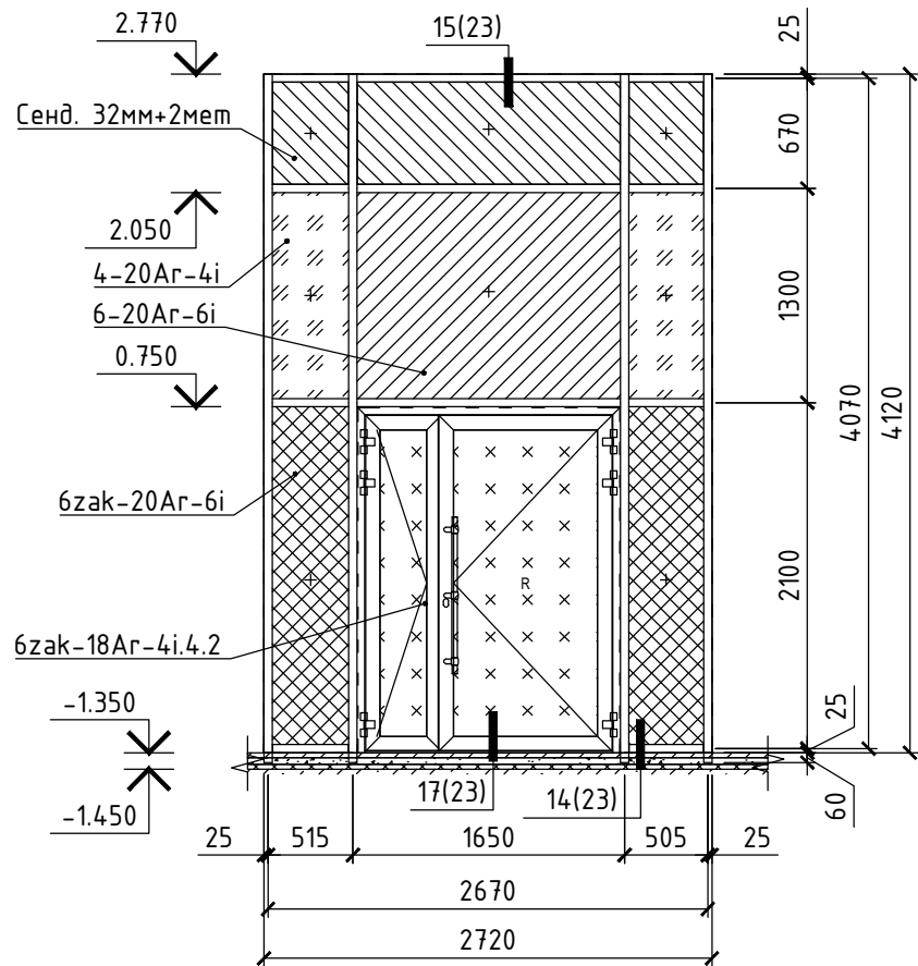
Витраж ВВ-3.2 (1 шт.)
