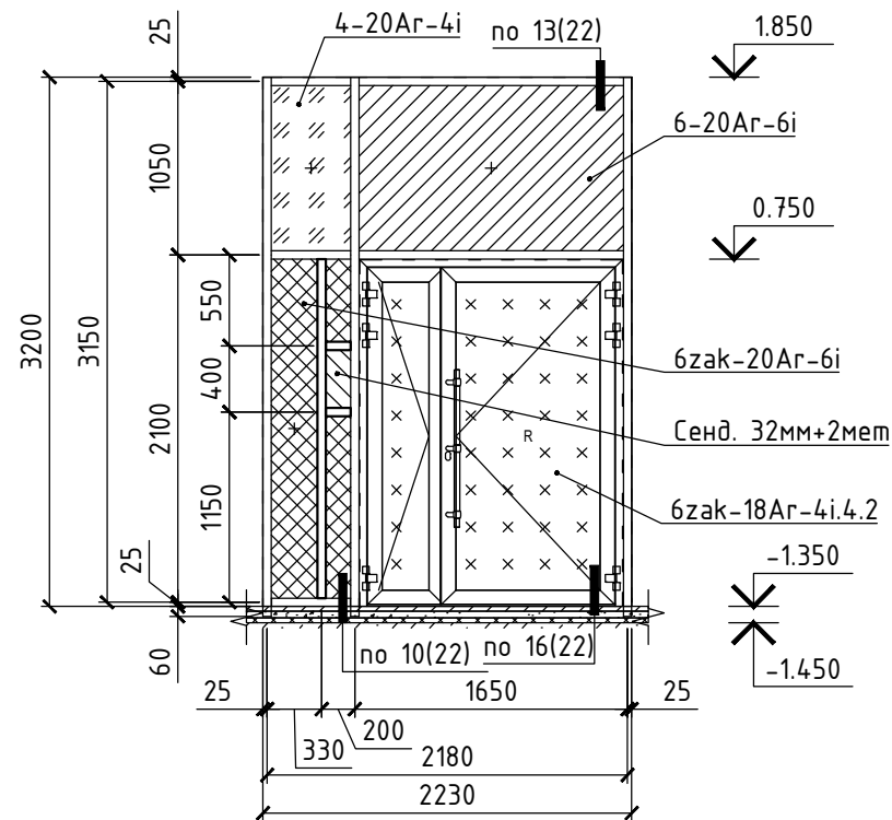
Витраж ВН-1.2 (1 шт.)
