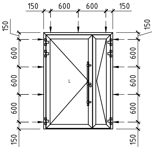
Схема крепления дверного блока
