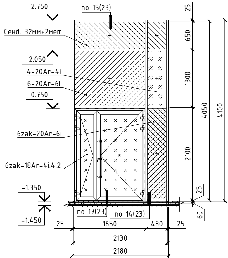
Витраж ВВ-4.1 (1 шт.)
