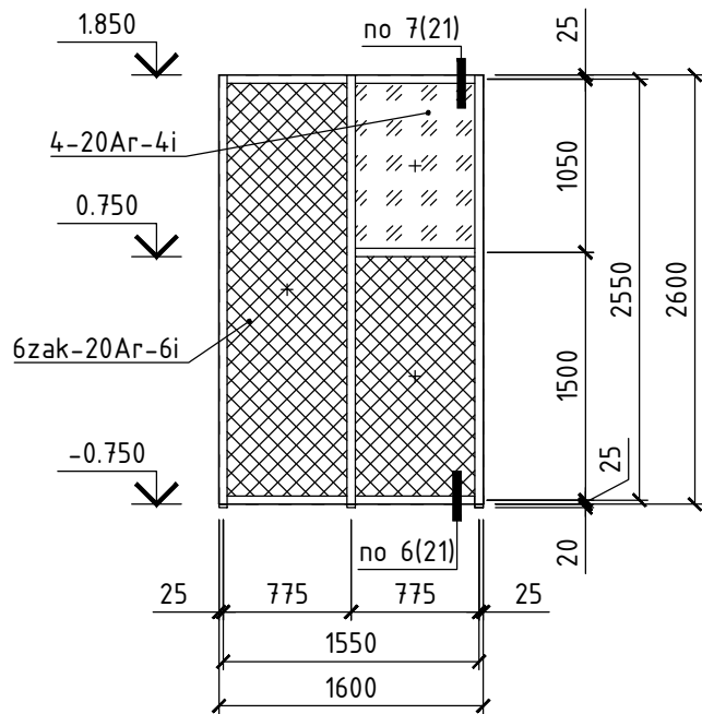
Витраж ВН-3.1 (1 шт.)
