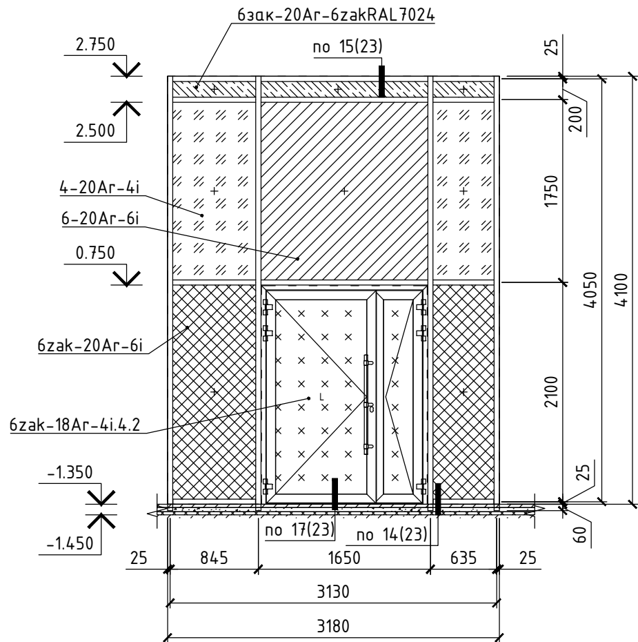
Витраж ВВ-4.2 (1 шт.)
