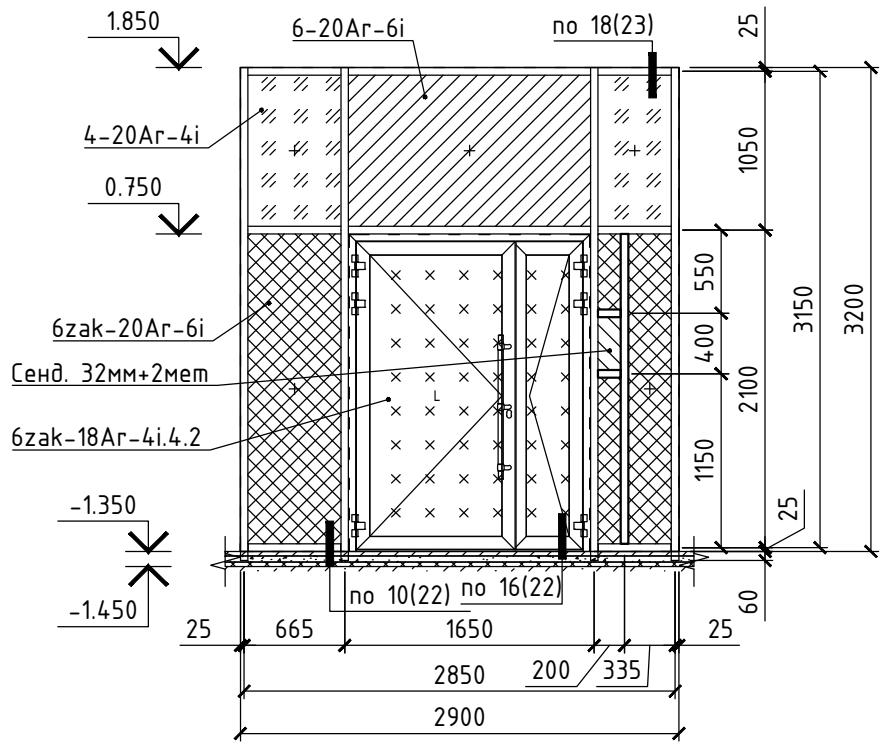
Витраж ВН-4.7 (1 шт.)
