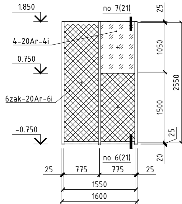
Витраж ВН-1.3 (1 шт.)
