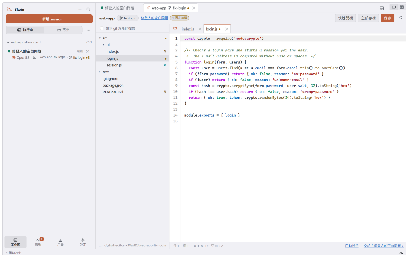
圖 9-4：編輯器是工作區的一個分頁，排在它那個 session 的分頁後面，標示「專案 分支」。左邊的檔案樹，檔名旁是 git 的狀態；開了兩個檔案，login.js 有還沒存的變更；標題旁說明有 1 個未存檔
