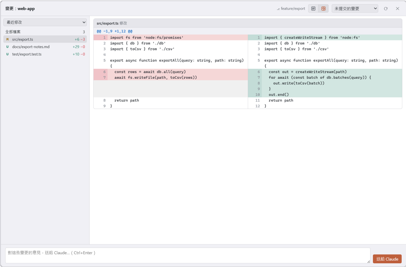
圖 10-3：左右對照：選了一個檔案，左邊是修改前、右邊是修改後
