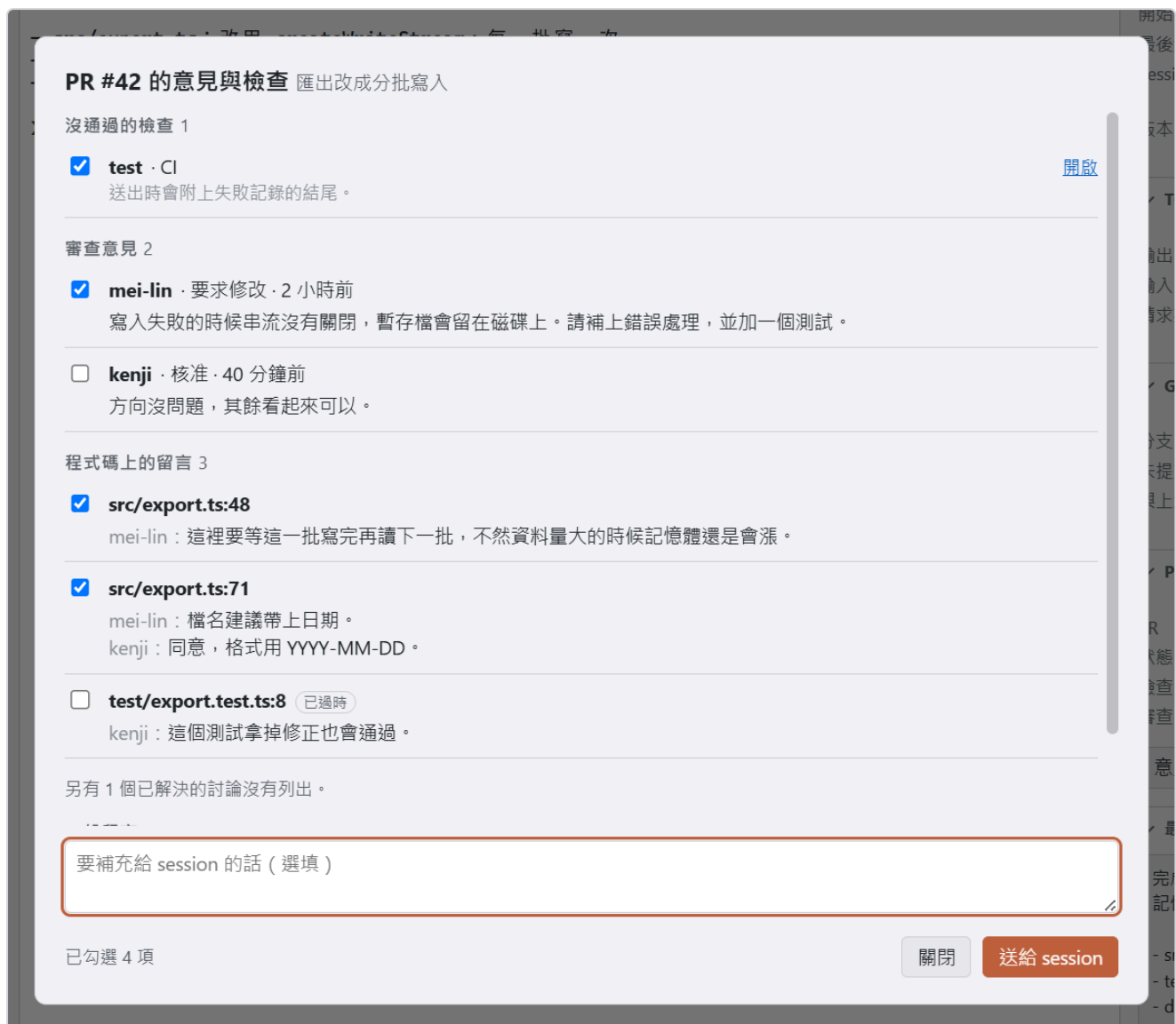
圖 11-6：「意見與檢查」對話框：沒通過的檢查、審查意見、程式碼上的留言各一組，每一項前面可以勾選，下方可以補充說明
