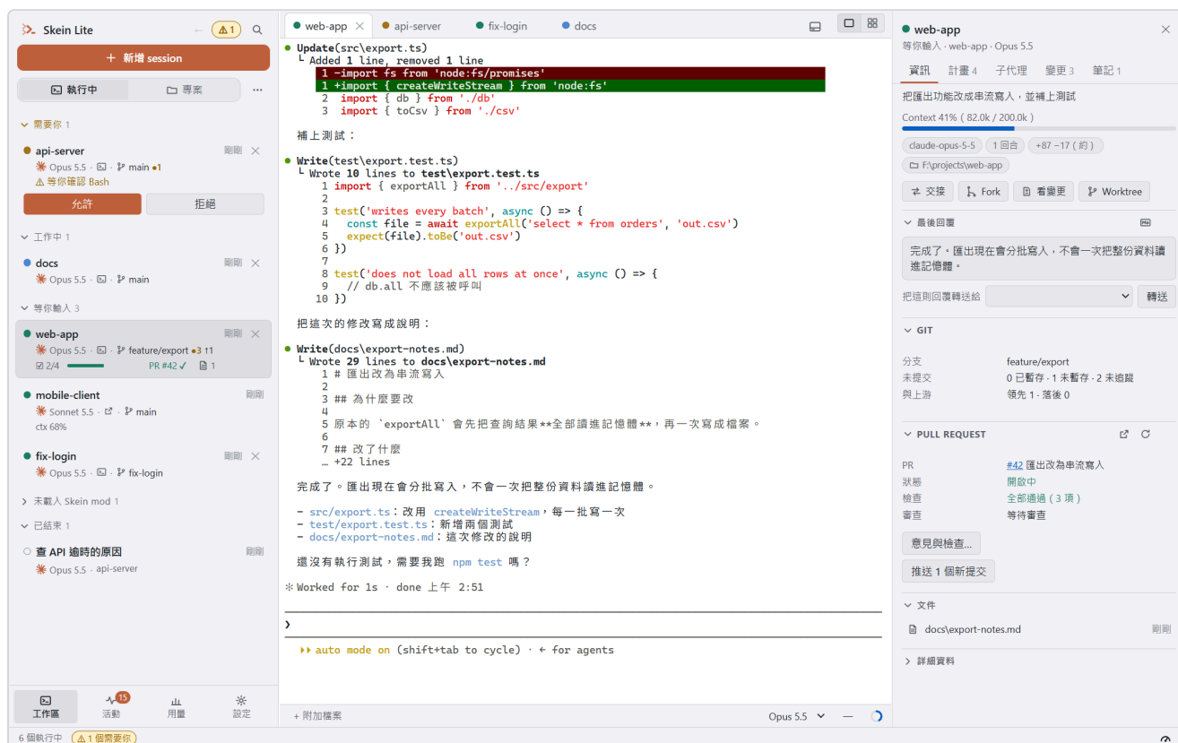
圖 1-1：主畫面全貌：左側清單有四個不同狀態的 session，中間是終端機，右側是資訊面板，下方是狀態列
