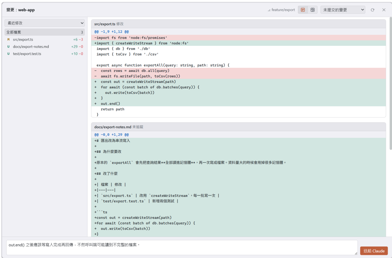
圖 10-1：diff 檢視：左邊是檔案清單（上方是排序選單，標示新增、修改、刪除），右邊是選到的檔案的內容，右上角是顯示方式的兩個圖示，下方是意見輸入框
