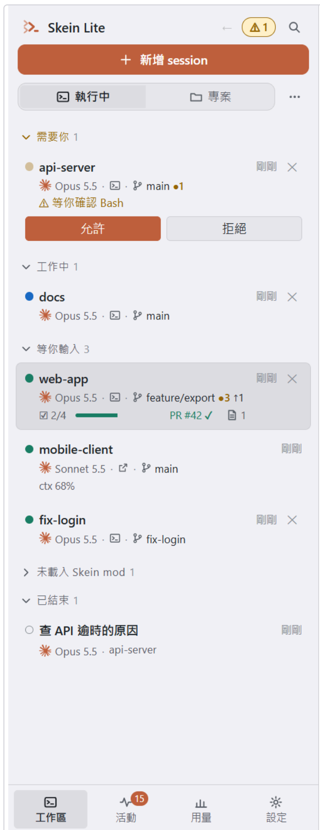
圖 3-2：左側清單的特寫：每列兩行，第二行依序是程式和模型、來源、資料夾、分支；「未載入 Skein mod」的分組是收合的
