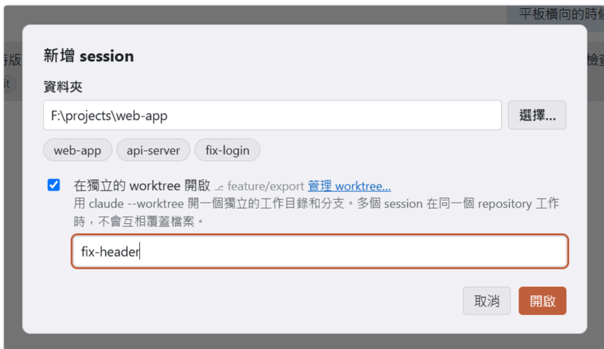
圖 9-1：新增 session 對話框，勾選了 worktree 並輸入名稱
