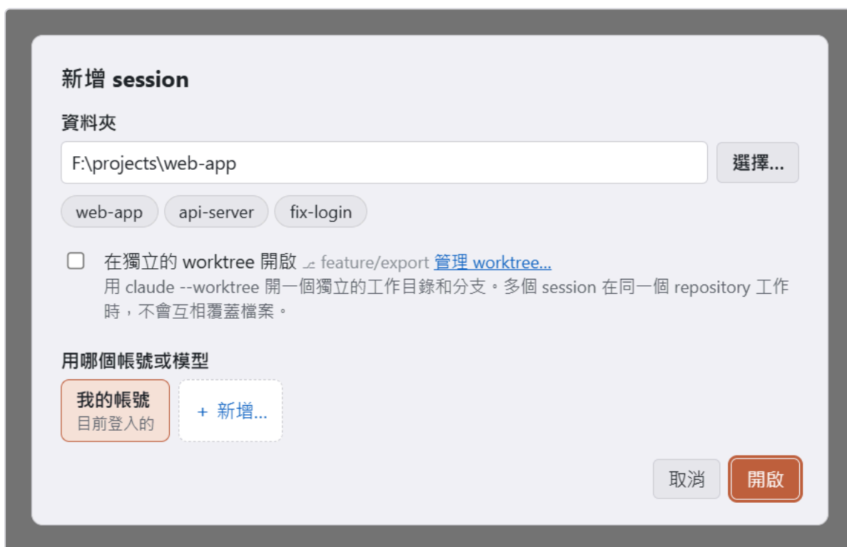
圖 4-1：新增 session 對話框：資料夾欄位、「在獨立的 worktree 開啟」的選項、「用哪個帳號或模型」
