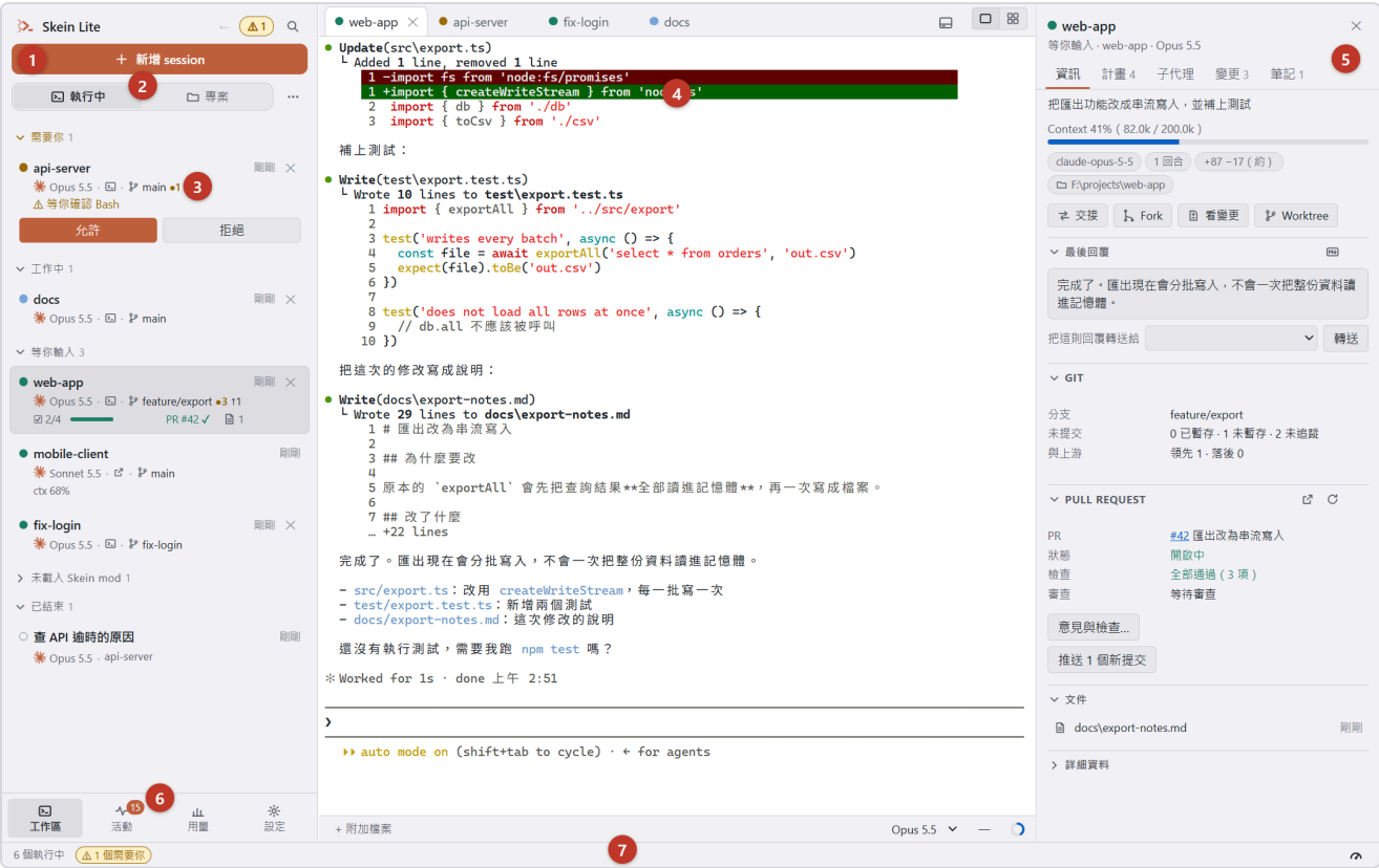
圖 3-1：主畫面，加上編號標示：① 新增 session ② 清單切換 ③ 左側清單 ④ 終端機區 ⑤ 右側面板 ⑥ 頁面切換 ⑦ 狀態列
