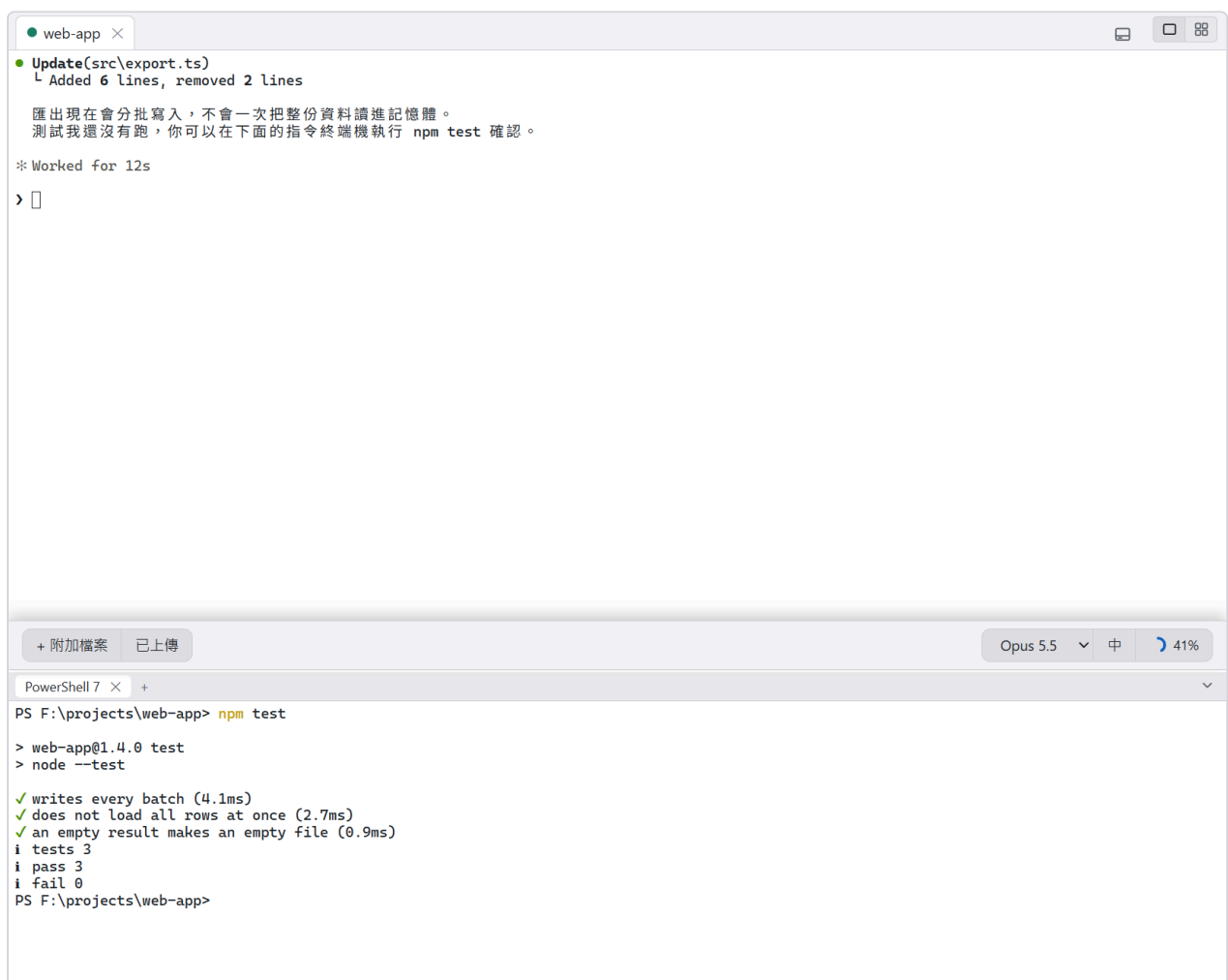
圖 4-6：指令終端機：上面是 session 的終端機，下面是自己下指令的地方，這裡剛跑完 npm test
