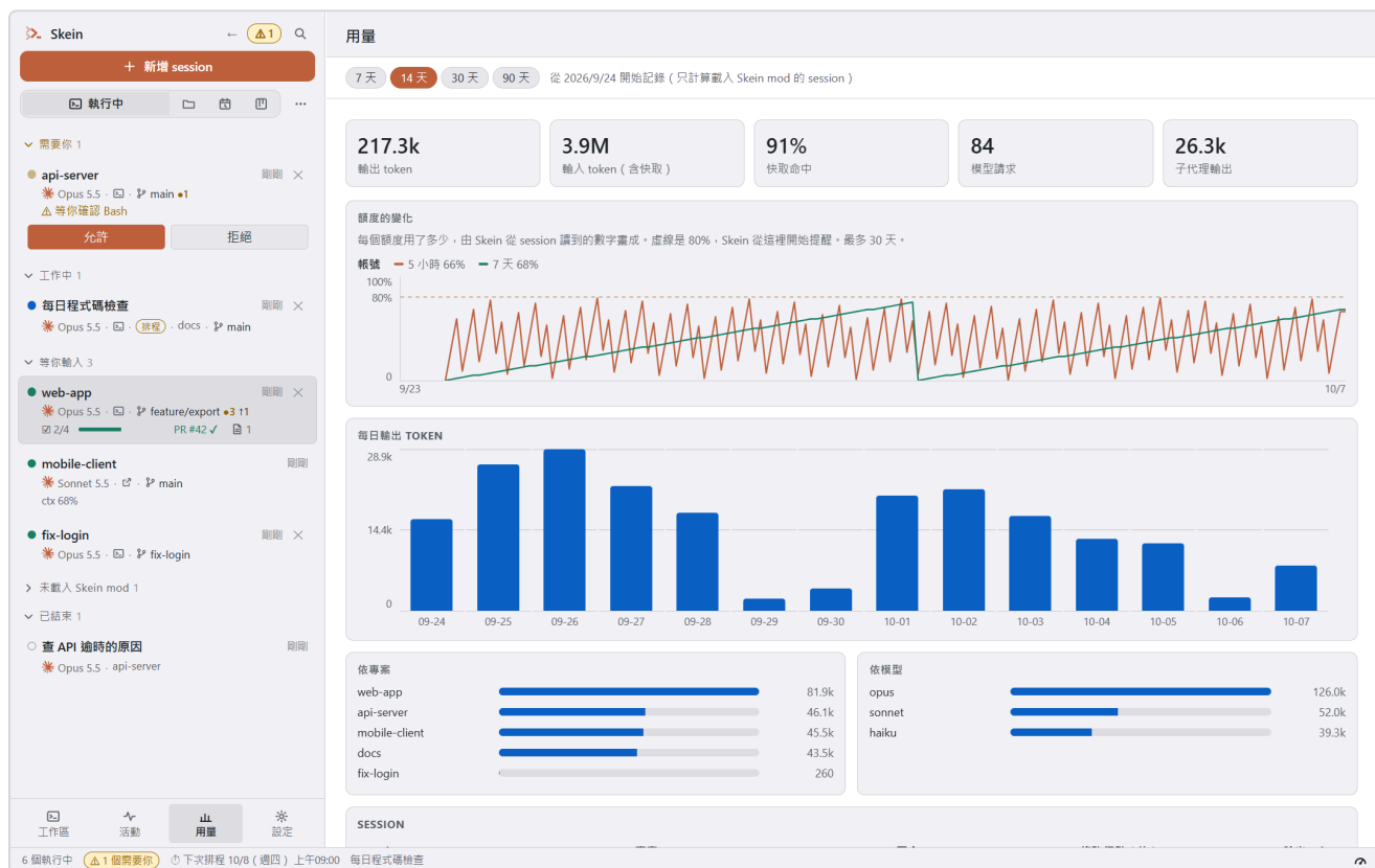
圖 14-1：用量頁：上方的時間範圍、五個總計數字、額度的變化、每日輸出 token 的長條圖、依專案和依模型的統計
