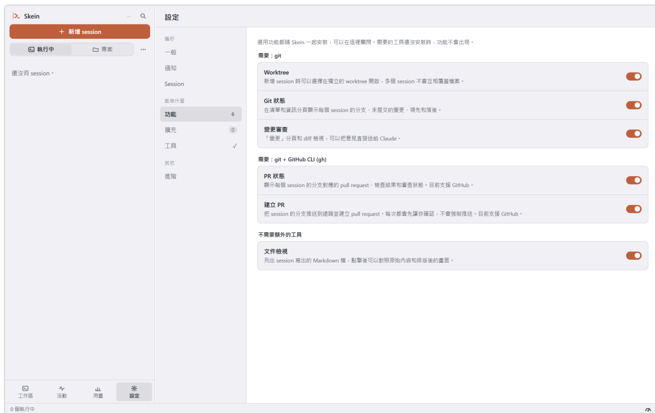
圖 9-0：設定的「功能」分類：Worktree、Git 狀態、變更審查、PR 狀態、建立 PR 五個開關，以及不需要 git 的文件檢視
