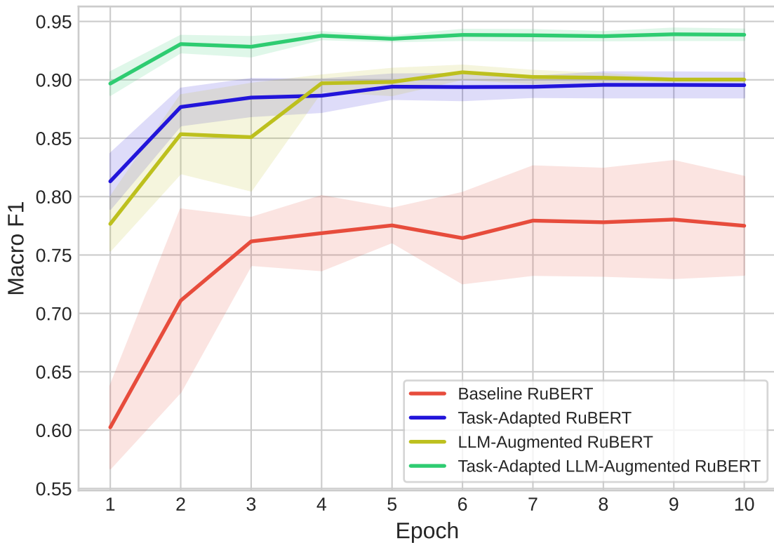
Validation Macro F1
