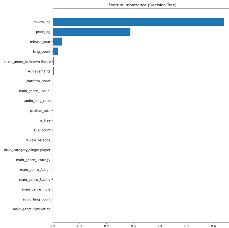
圖 13 Decision Tree 特徵重要性圖
