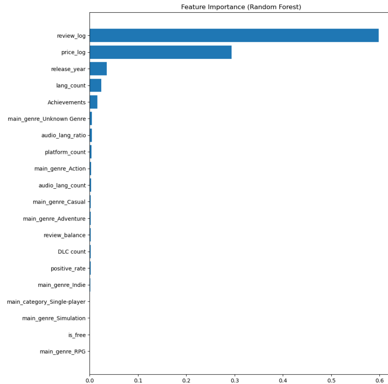
圖 14 Random Forest 特徵重要性圖
