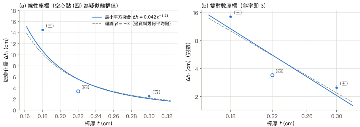
圖 5： \Delta h_i 對棒厚 t 的關係。藍線為乘幂擬合，灰色虛線為理論 \beta = -3 ；空點(四) 偏離預測達 43%。
