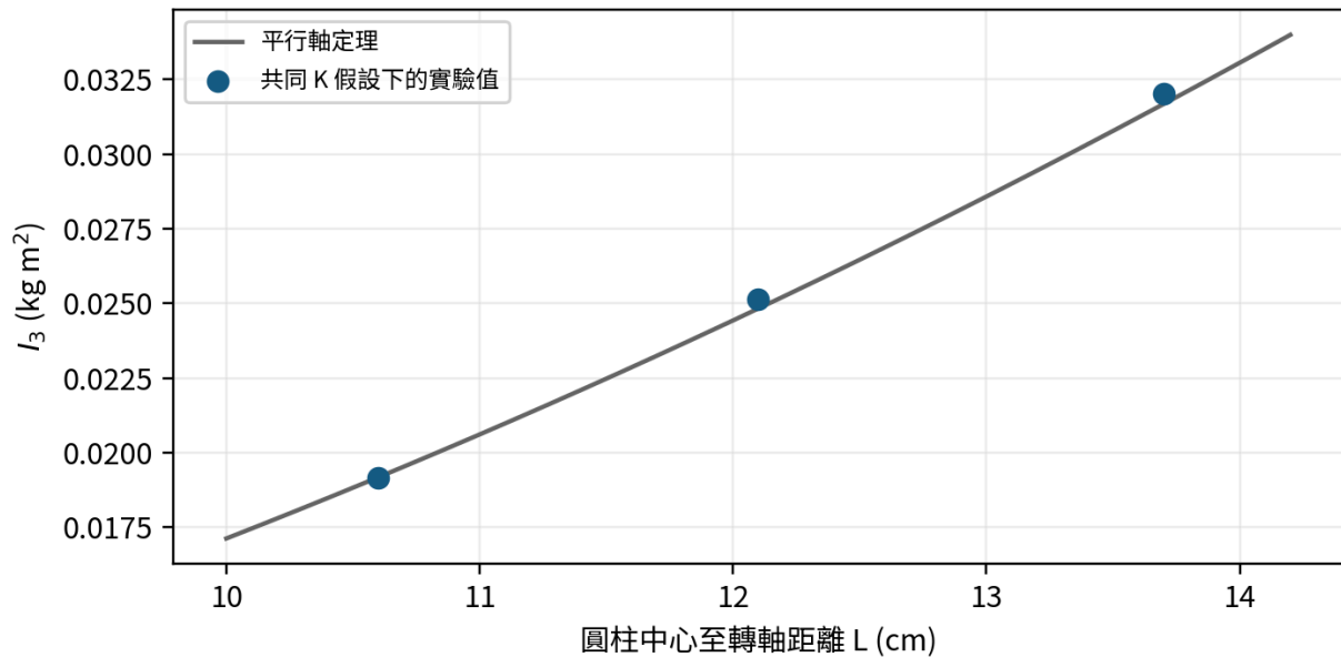
圖2 兩圓柱轉動慣量與中心距離。曲線直接取平行軸定理的理論式，並非用三點硬套二次曲線。
