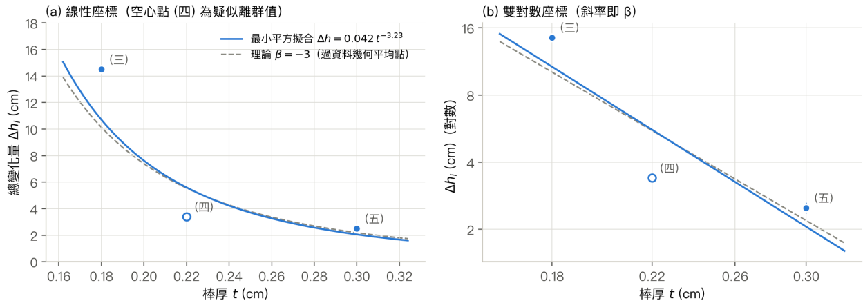
圖 5： \Delta h_i 對棒厚 t 。藍線為乘冪擬合，灰色虛線為理論 \beta = -3 ；空心點為棒 (四)。
