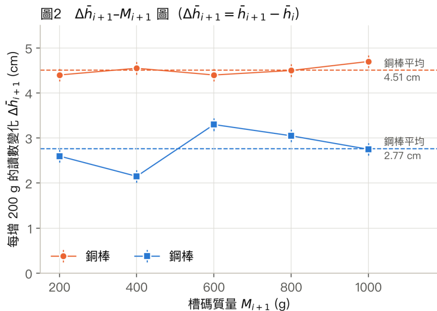
圖 2：每增加 200 g 時讀數的變化 \Delta\bar{h}_{i+1} 。虛線為平均值，誤差棒 \pm 0.14 \text{ cm} 。
