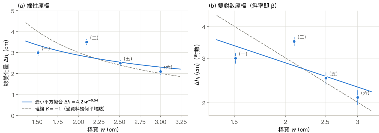
圖 4 : \Delta h_i 對棒寬 w 。藍線為乘冪擬合，灰色虛線為理論 \beta = -1 。
