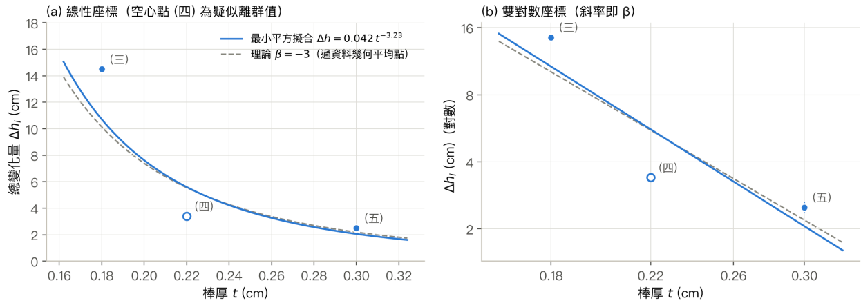
圖 5：鋼棒的 \Delta h_i 對棒厚 t 。(a) 線性座標，(b) 雙對數座標，斜率即 \beta ；藍線為乘幂擬合，灰色虛線為理論 \beta = -3 ，空心點為棒 (四)。
