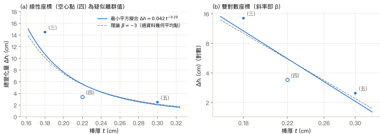
圖 5 : \Delta h_i 對棒厚 t 的關係。藍線為乘冪擬合，灰色虛線為理論 \beta = -3 ；空心點(四) 偏離預測達 43%。
