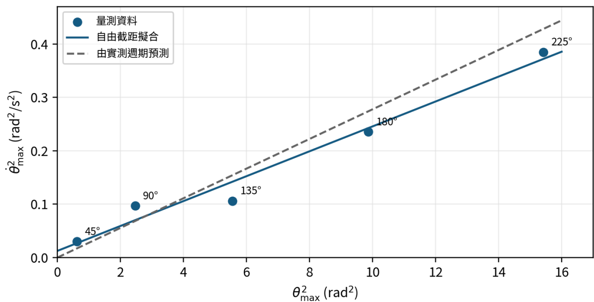
圖1 最大角速度平方與最大扭角平方。實線為未強制通過原點的最小平方法；虛線由 T_0 = 37.70 s 預測。
