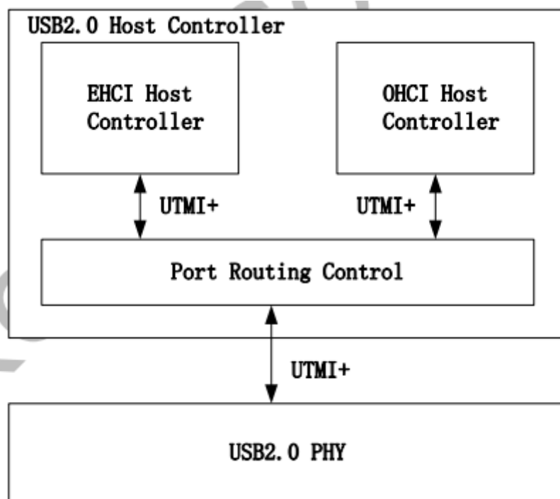
图 1-1 USB 2.0 Host 控制器框图
