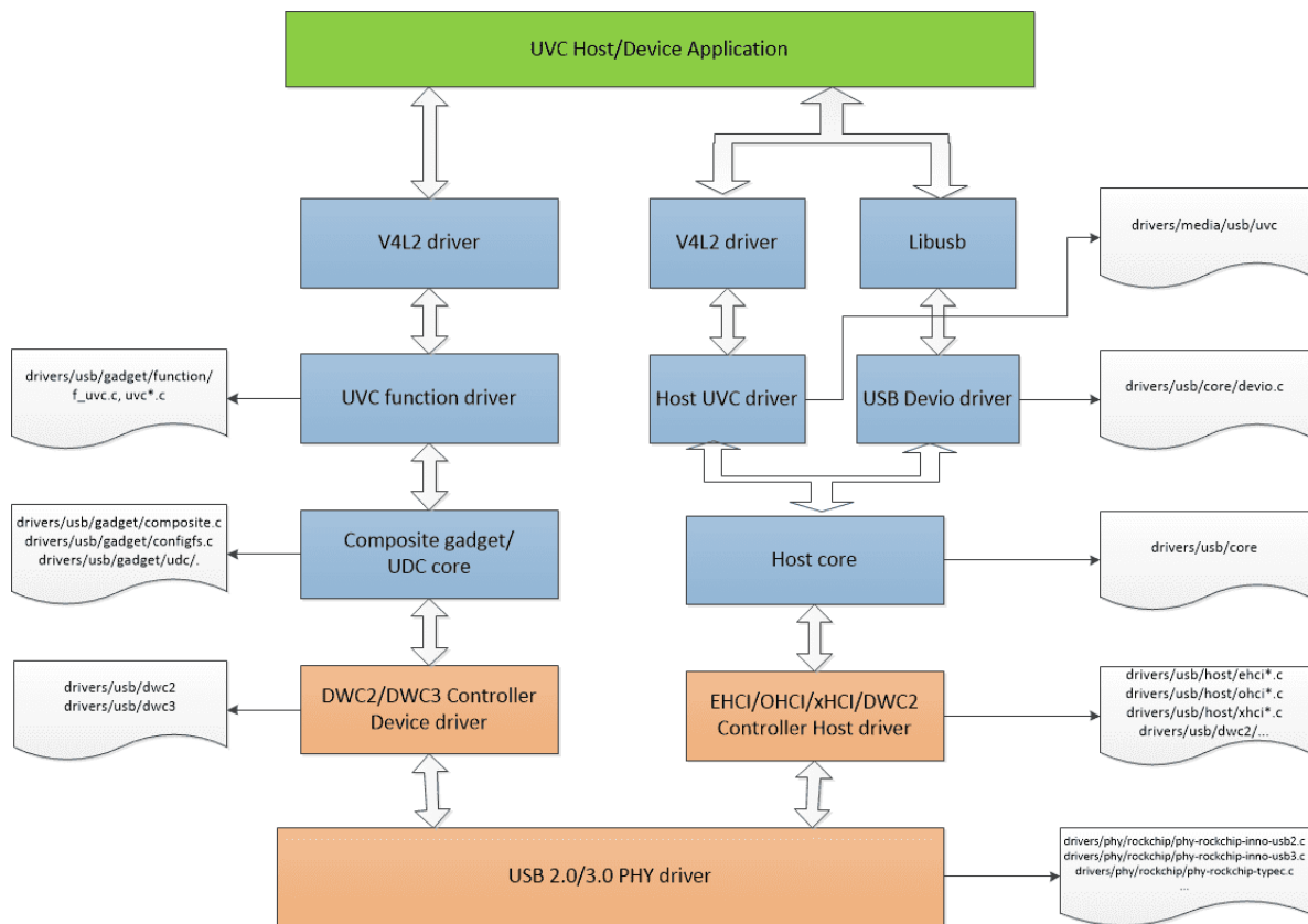
图 1 Linux UVC 通信流程
