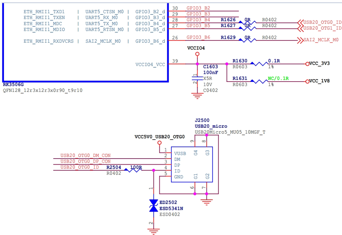
图 2-16 USB OTG_ID GPIO 硬件电路
