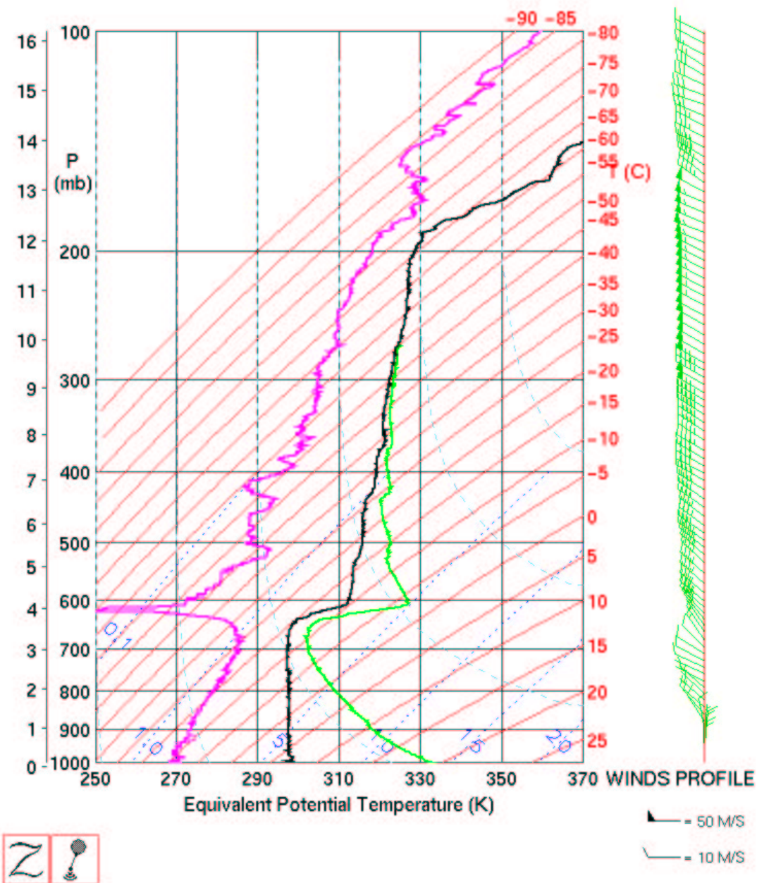
Figura 14: Theta-Plot del radiosondaggio effettuato a Campoformido (WMO 16044) il 28 ottobre 2002 alle ore 12 UTC. La costanza della \Theta_e e di q indicano come fino a 3397 m s.l.m. l'atmosfera segua un'adiabatica secca. Segue uno strato d'inversione spesso ben 800 m.
