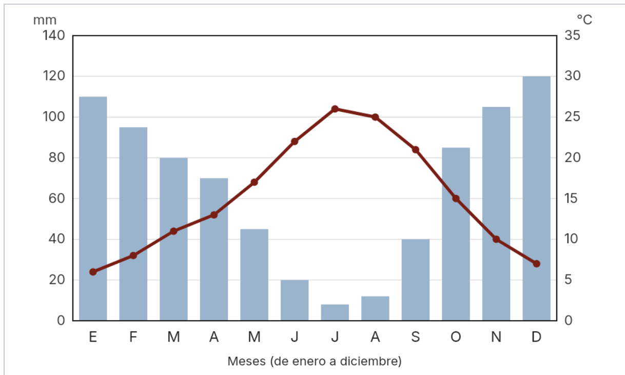
Climograma de Valdeloma: precipitaciones (barras, mm) y temperatura media (línea, °C) de cada mes
