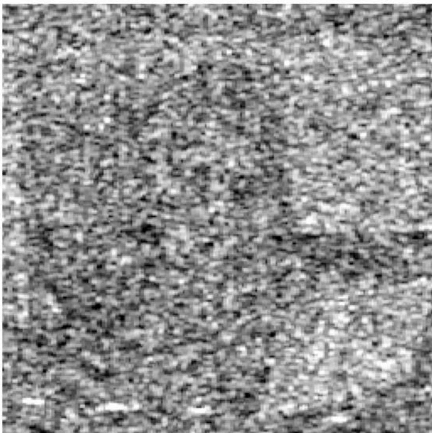
SAR (scene 84)
