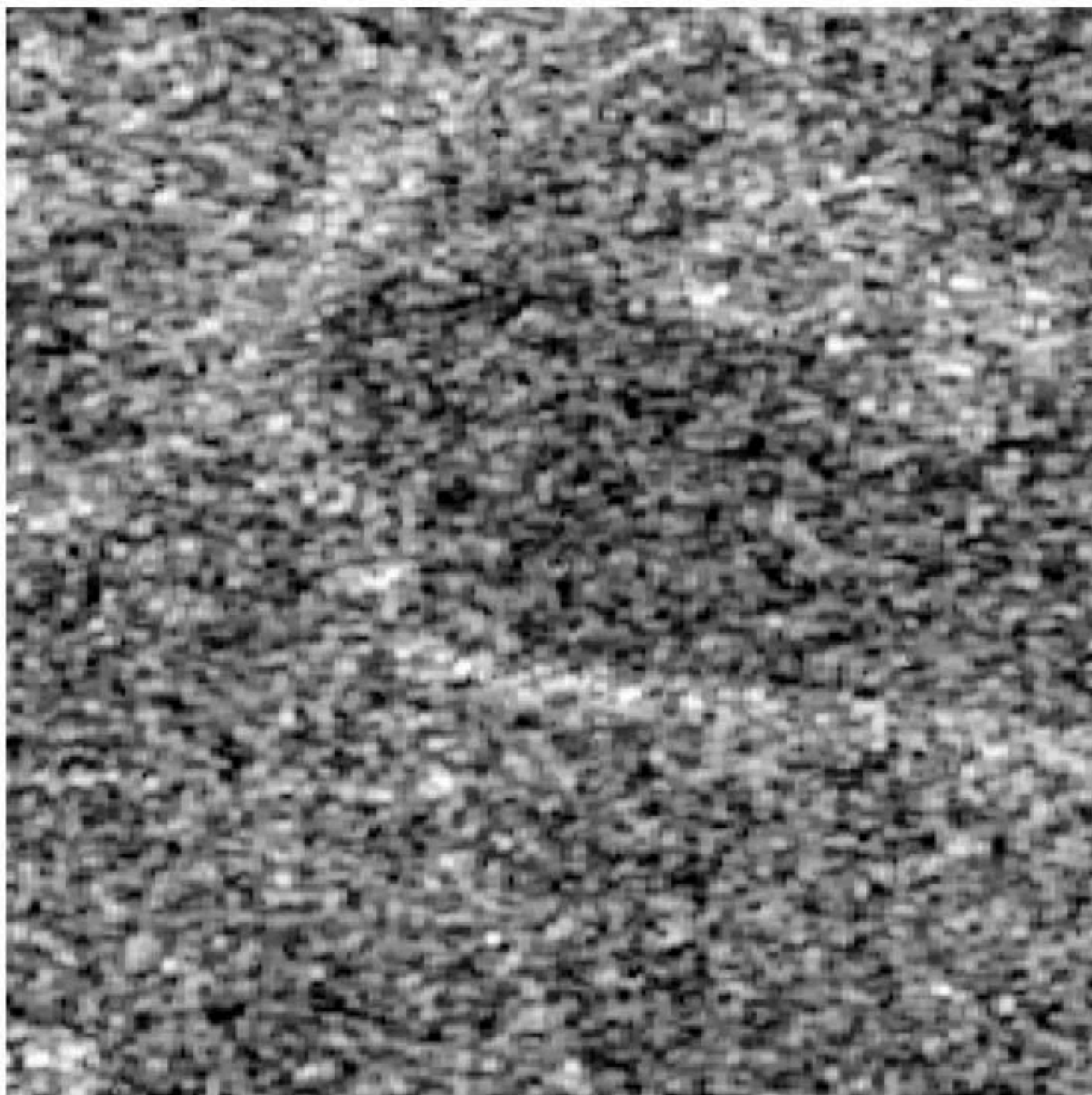
SAR (scene 84)
