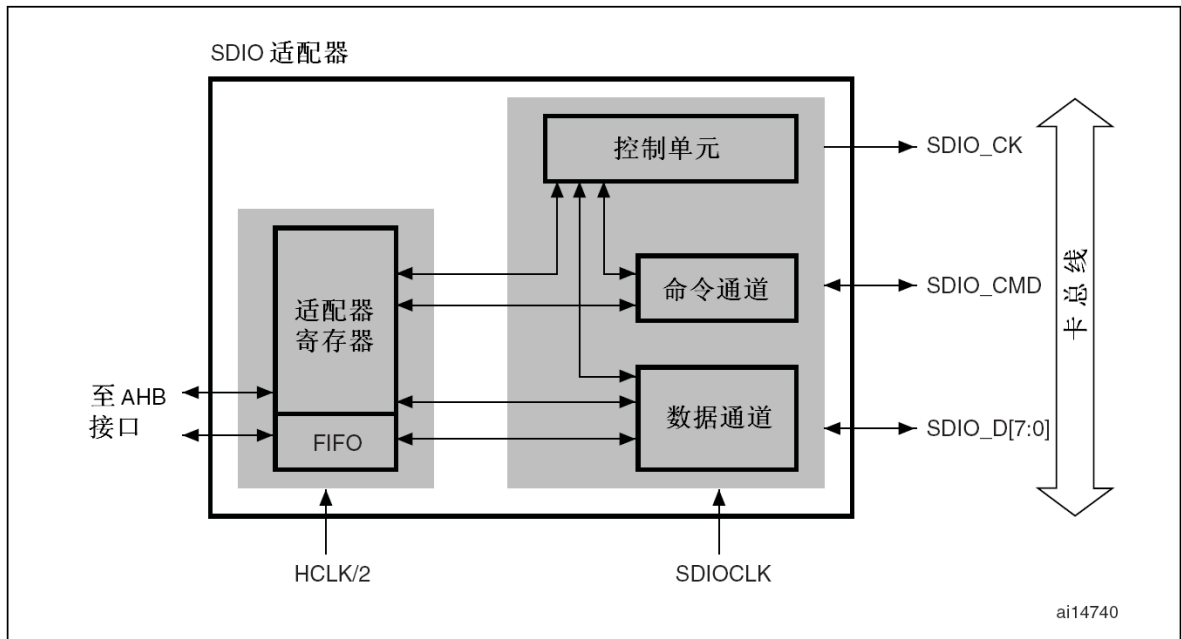
图185 SDIO适配器
