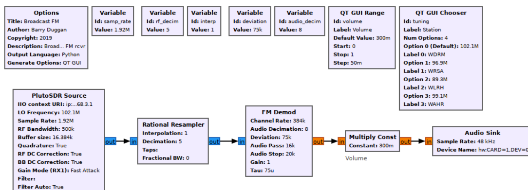
FIGURE 1 – Exemple de récepteur FM
