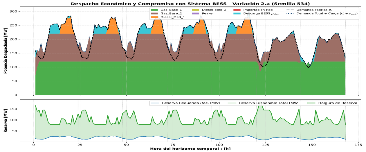
Figura 3: Despacho económico apilado y reserva operativa horaria incorporando el sistema de almacenamiento de energía (Variación 2.a).
