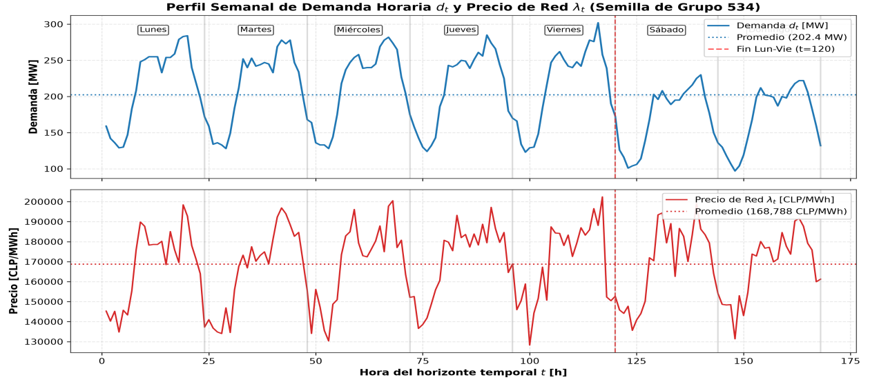
Figura 1: Perfiles semanales de demanda horaria d_t y precio de importación de la red \lambda_t .
