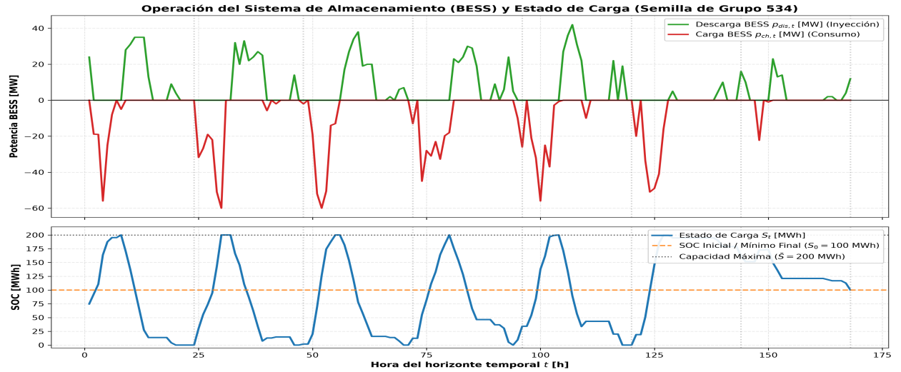
Figura 4: Ciclos de carga, descarga y evolución del estado de carga ( S_t ) de la batería (Semilla 534).
