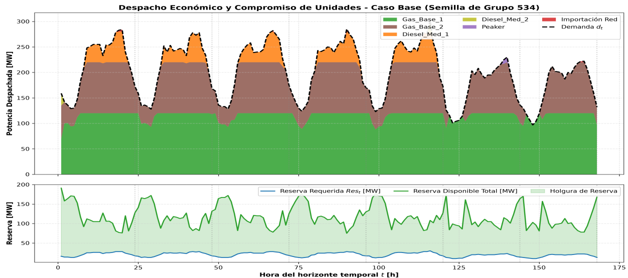
Figura 2: Despacho económico apilado y reserva operativa horaria en el Caso Base.
