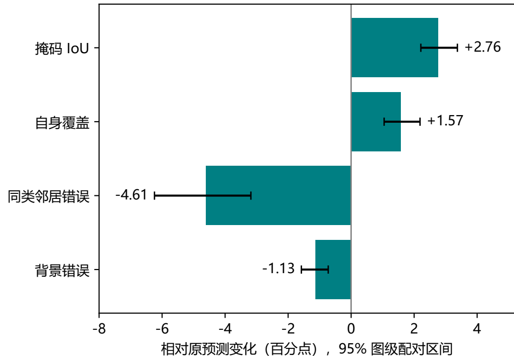
只换系数：高组像素变化
