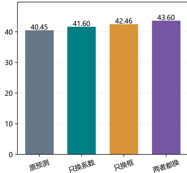
整图 Mask AP
