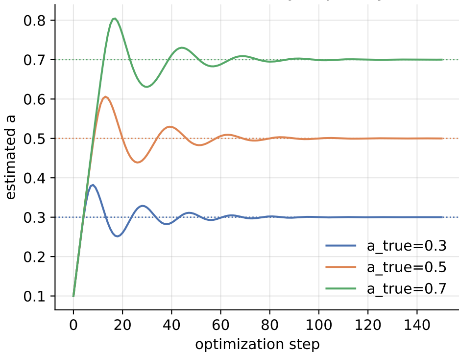
Parameter recovery trajectory
