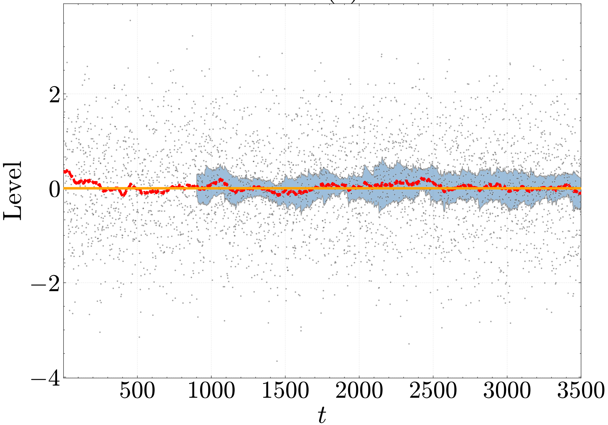
AR(1)
