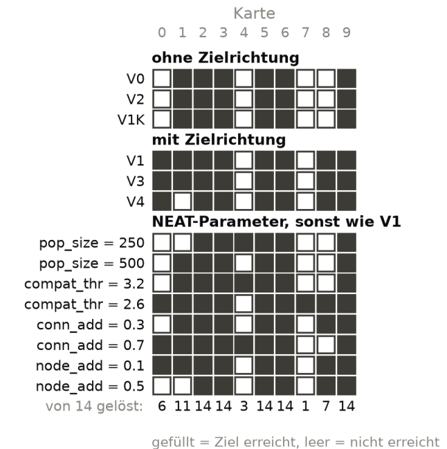
Abbildung 1: Alle 14 Konfigurationen gegen die zehn Karten der Hauptmessung, ein Quadrat je Lauf. Fünf Karten lösen alle Konfigurationen, zwei fast keine. Die Zeilen unterscheiden sich deutlich weniger als die Spalten. V0 und V2 lösen dieselben Karten, V1 und V3 ebenfalls.
