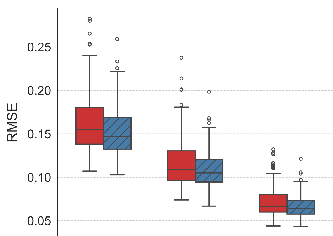
rho
