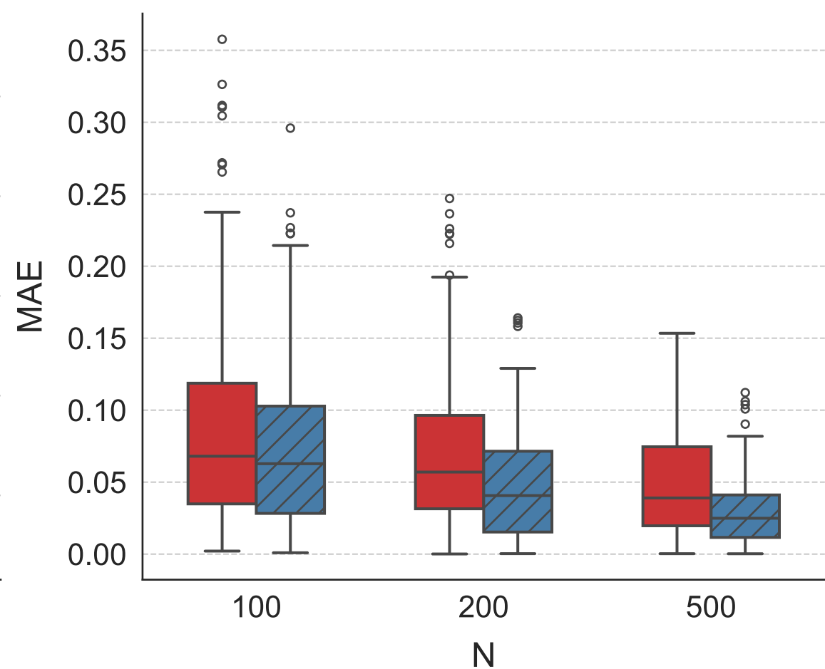
rho
