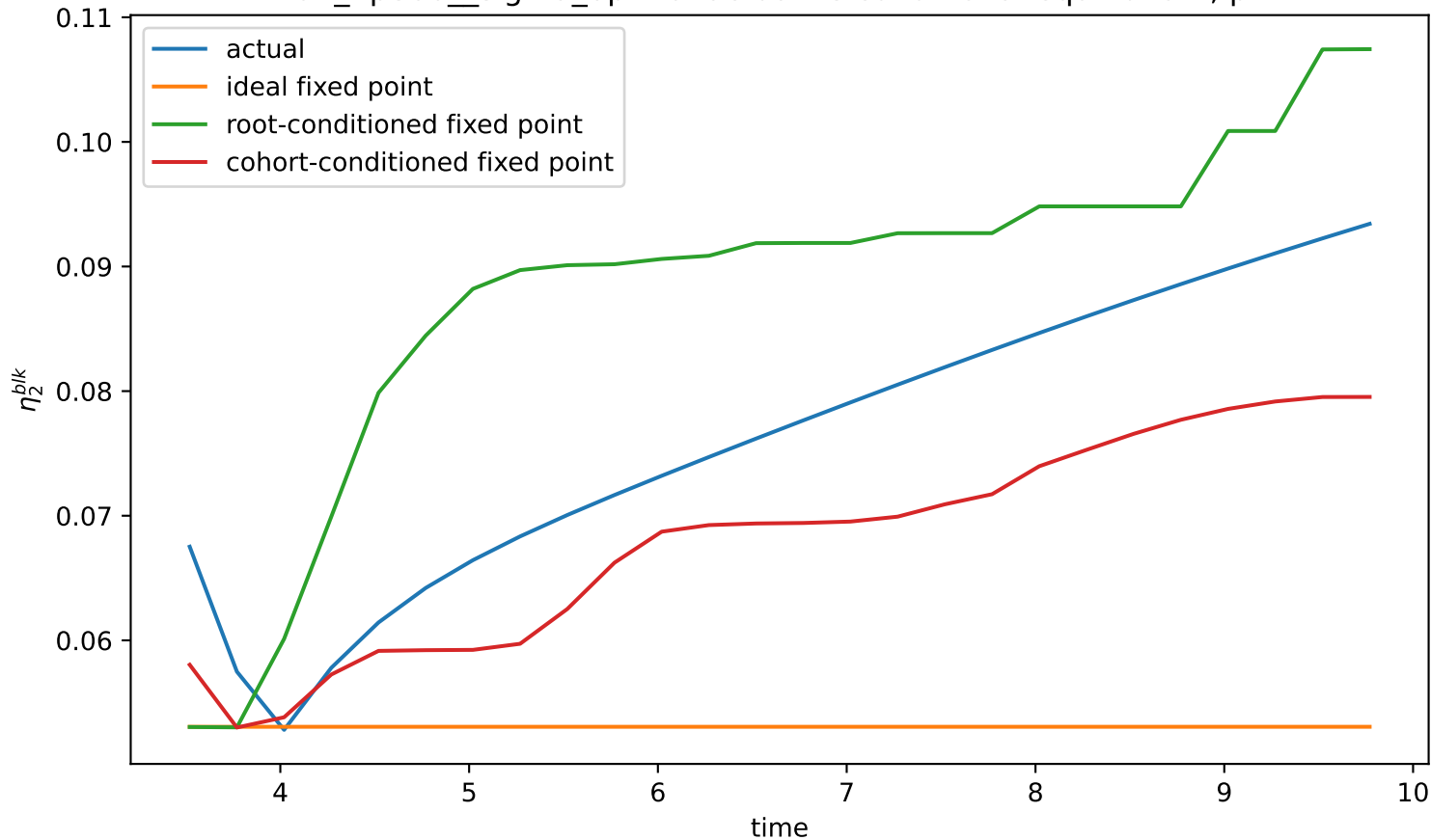
mu2_1p800_sigma_0p120: actual vs conditional equilibrium, p=2
