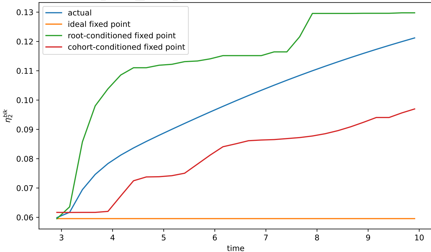
mu2_2p000_sigma_0p150: actual vs conditional equilibrium, p=2
