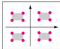
d. 16-QAM
