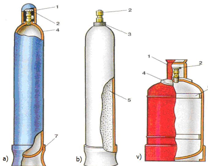
14.1 – rasm. Yuqori bosim ostida ishlovchi ballonlar:
