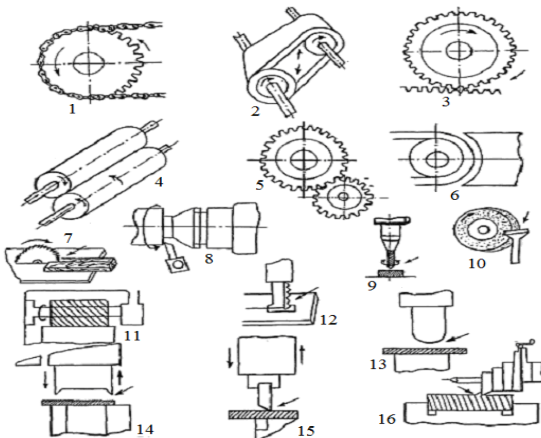
8.1 rasm. Mashina va mexanizmlarning xavfli joylari (o‘q chiziqlar bilan ko‘rsatilgan):
