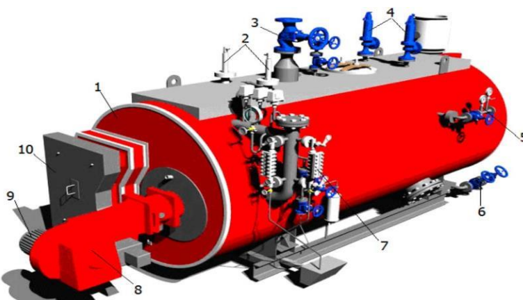
14.3 – rasm. Bug' hosil qilish qozoni:
