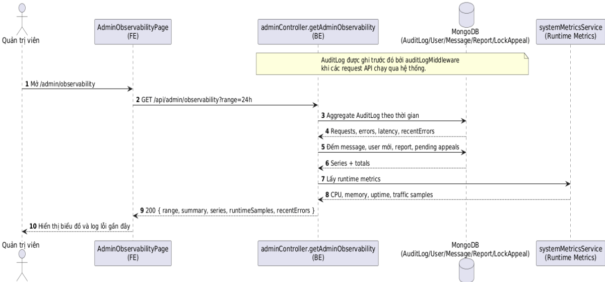
Hình 26. Lược đồ tuần tự Xem log hệ thống
