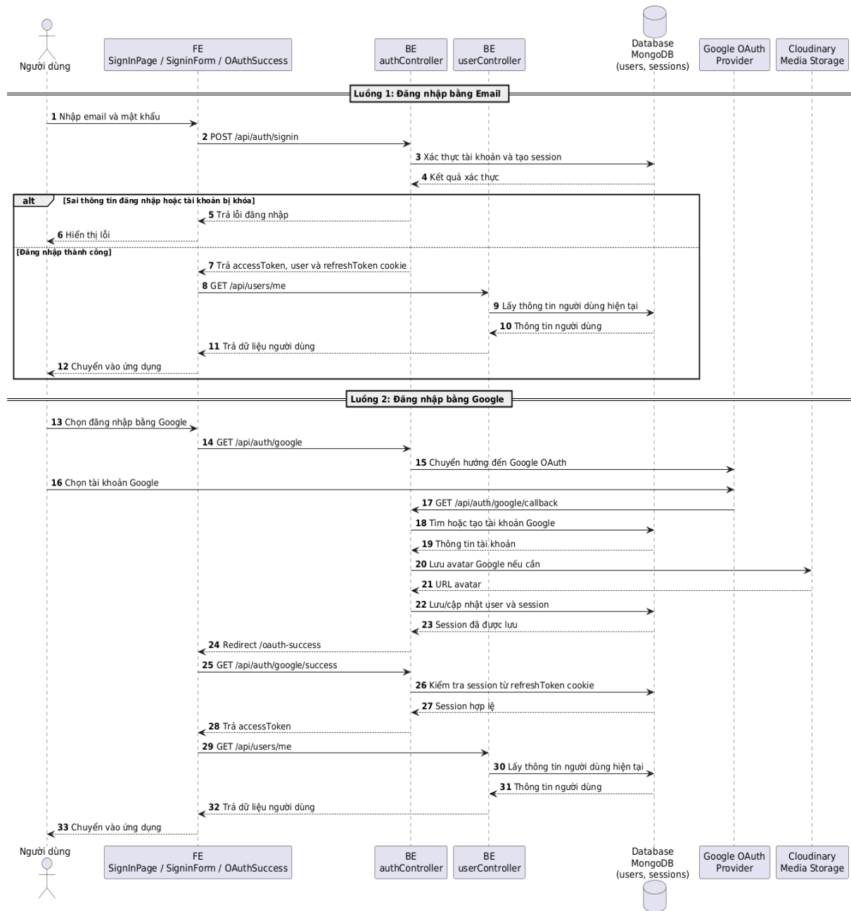
Hình 8. Lược đồ tuần tự Đăng nhập
