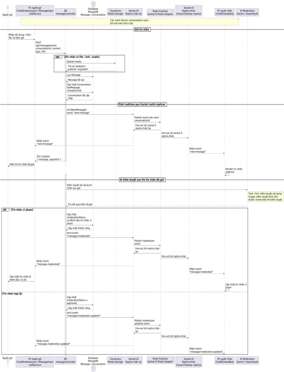
Hình 15. Lược đồ tuần tự Gửi và Nhận tin nhắn
