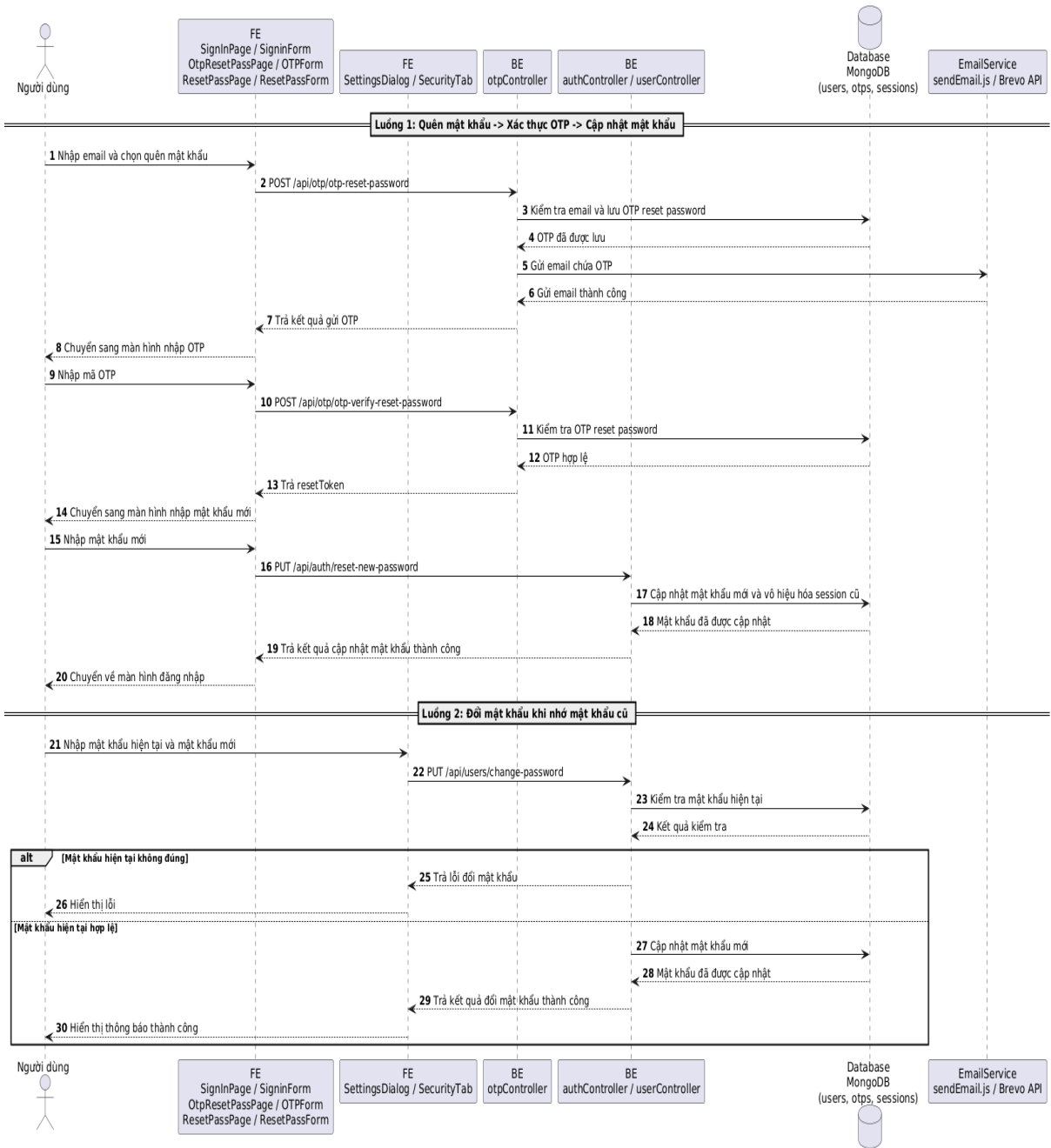
Hình 9. Lược đồ tuần tự Quên mật khẩu và Cập nhật mật khẩu
