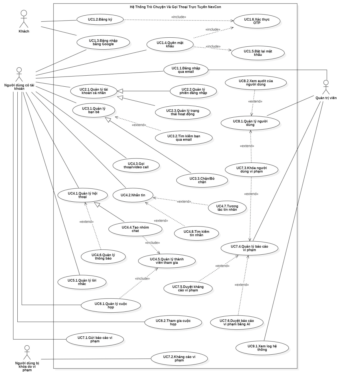
Hình 6. Biểu đồ chức năng
