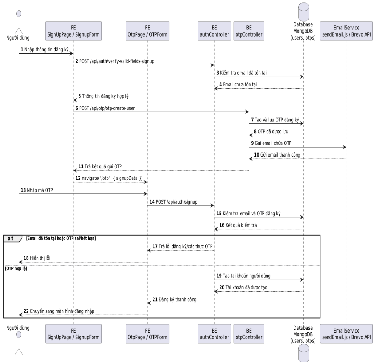
Hình 7. Lược đồ tuần tự Đăng ký tài khoản và Xác thực OTP
