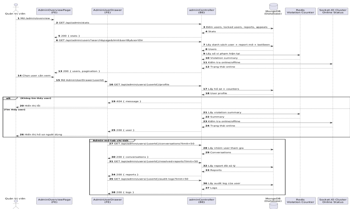
Hình 23. Lược đồ tuần tự Xem danh sách người dùng và chi tiết
