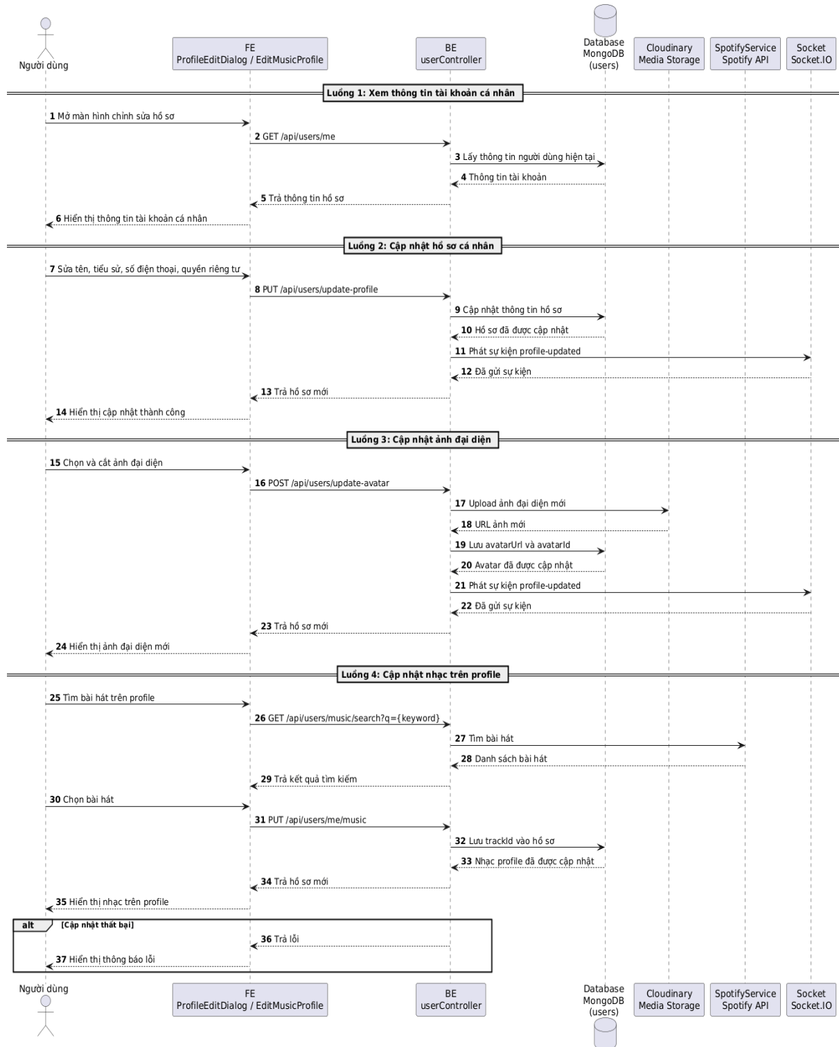
Hình 10. Lược đồ tuần tự Quản lý tài khoản
