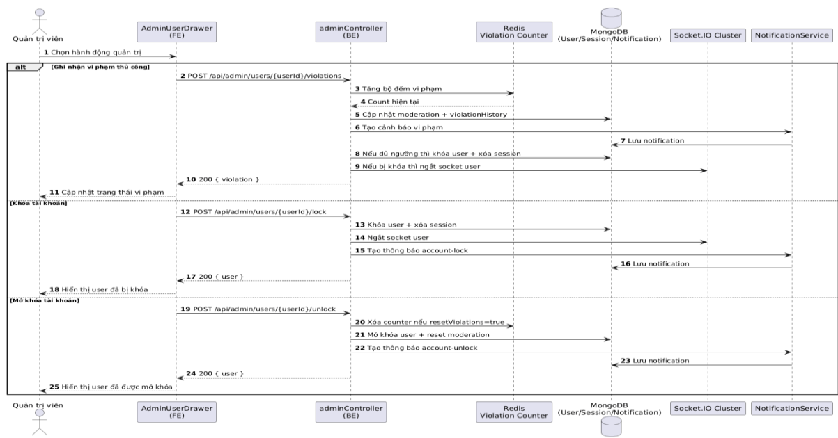
Hình 24. Lược đồ tuần tự Ghi nhận vi phạm, Khóa và Mở khóa tài khoản
