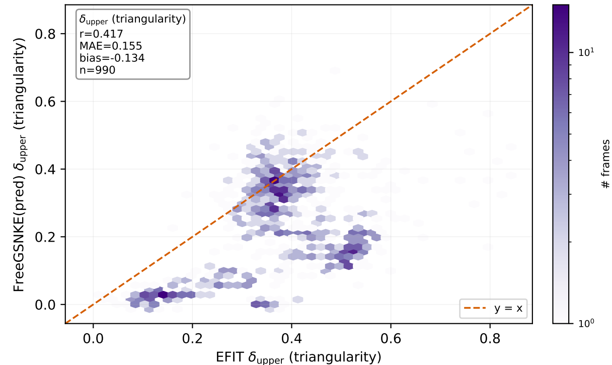
(d) Shape parity
