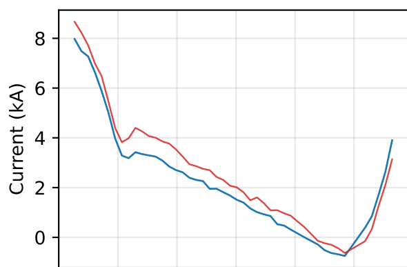
PF4 ( R^2=0.930 , RMSE=0.57 kA)
