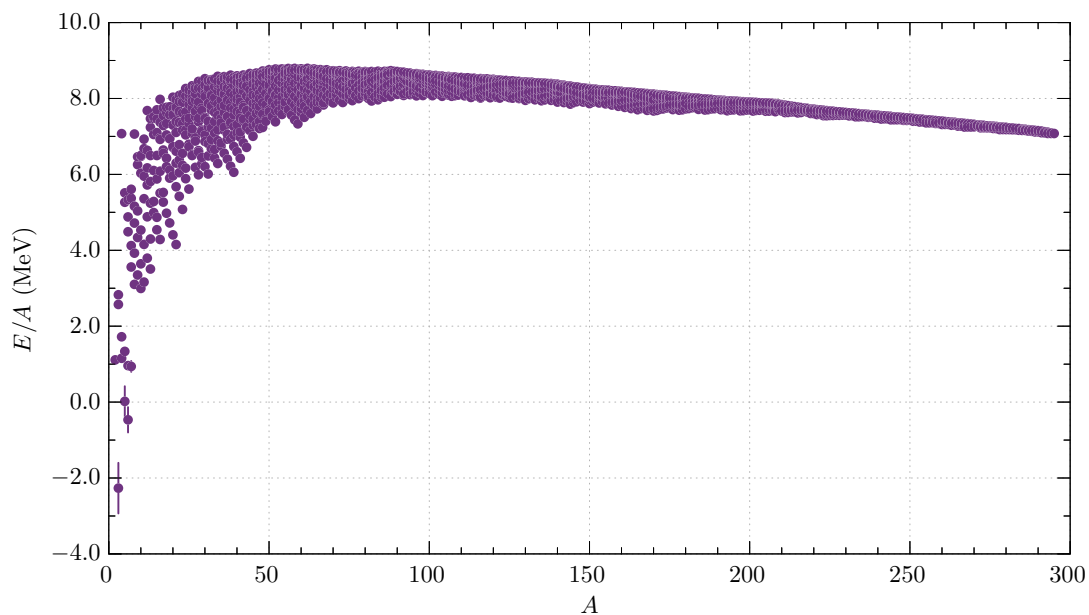
図1 質量数 A の関数として表した核子あたりの結合エネルギー E/A の実験値 [2]. ここでは Z や N は指定していないため、同位体や同重体は区別していない。
